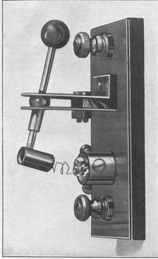
FIG. 17.—CRYSTAL DETECTOR.
