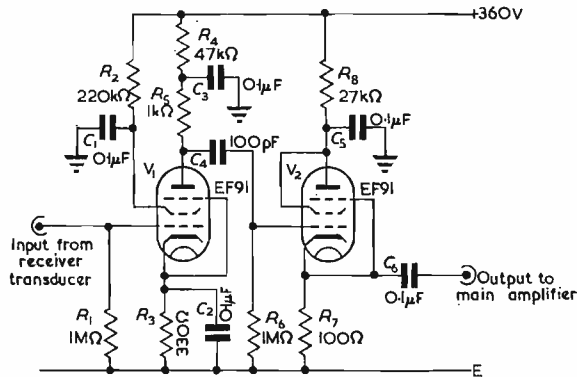
Fig. 12. Pre-amplifier
