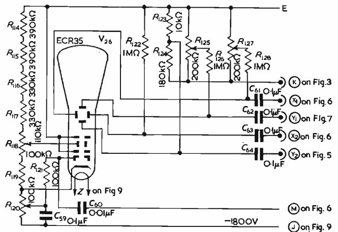
Fig. 8. Display unit
