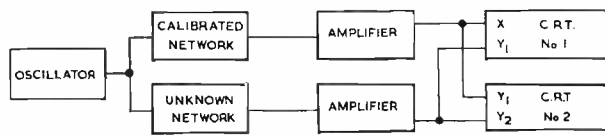
Fig. 3. The oscilloscope connexions
