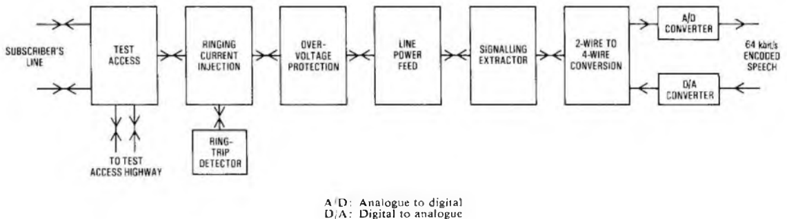
FIG. 6—Line-circuit structure
