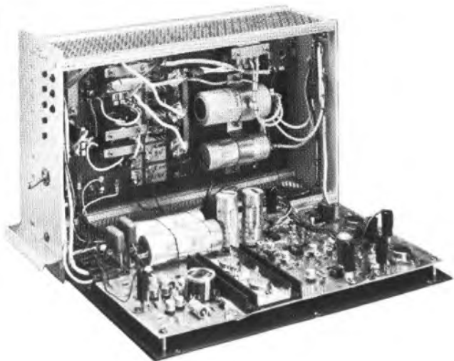
FIG. 2—DC-DC converter
