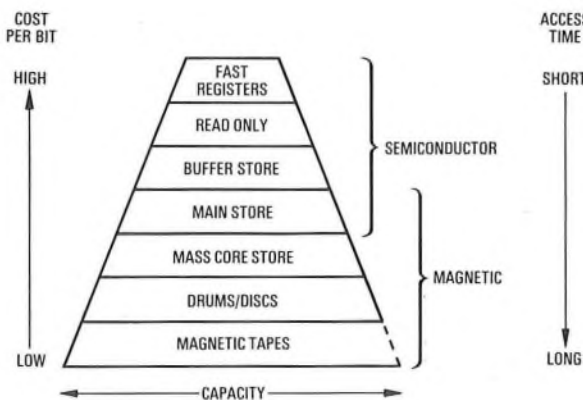
FIG. 1—Store hierarchy
