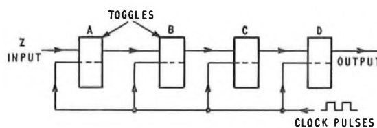
FIG. 2—Shift register
