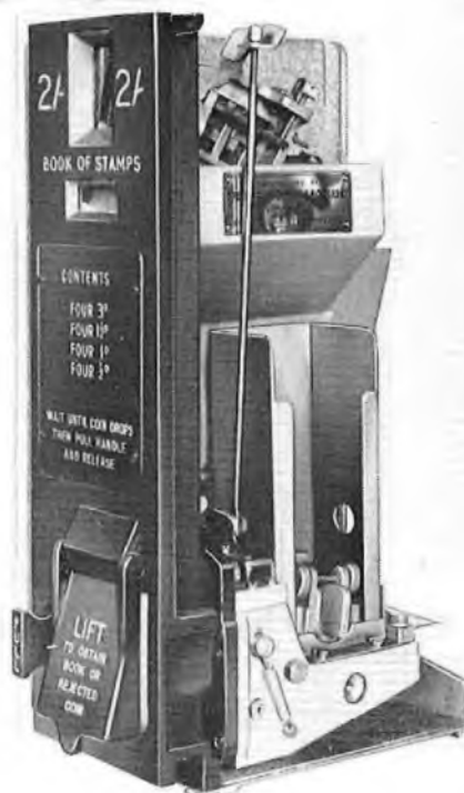
FIG. 2—2s. STAMP-BOOKLET MACHINE, TYPE F1
