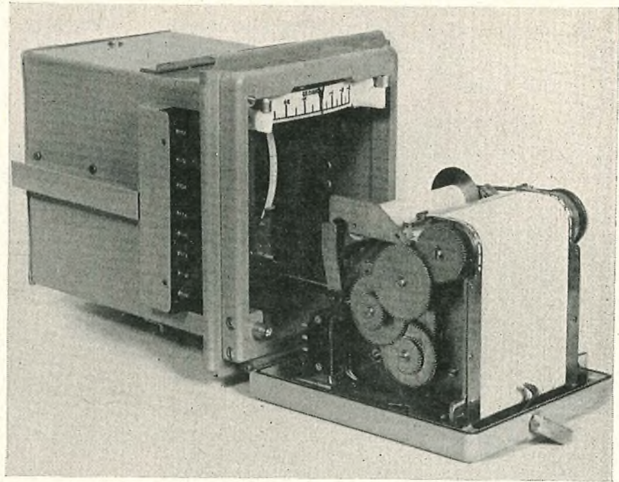
FIG. 3—DECIBELMETER NO. 28A/CTA
