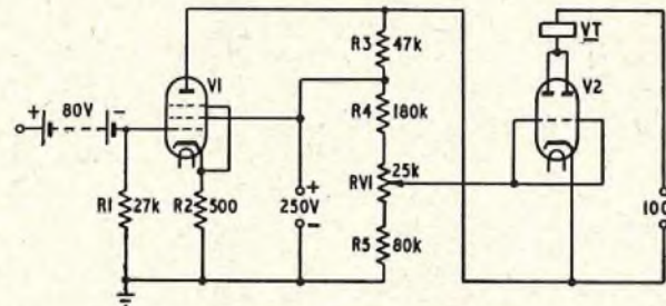
FIG. 6—VALVE-VOLTMETER CIRCUIT
