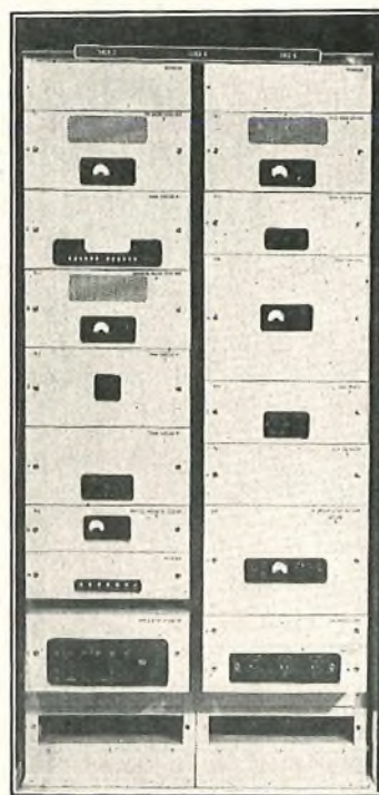
FIG. 7.—CLOCK B.
