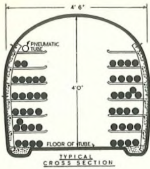
FIG. 3.—OLD PARCELS TUBE.
