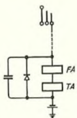
FIG. 9.—QUENCH CIRCUIT.
