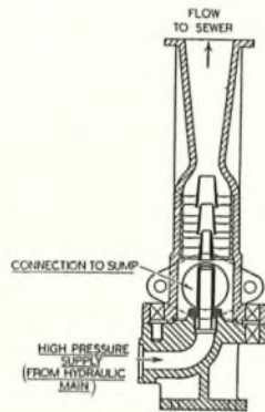
FIG. 20.—HYDRAULIC EJECTOR.
