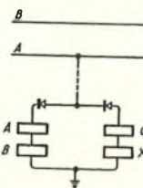
FIG. 8.—DISCRIMINATING CIRCUIT.
