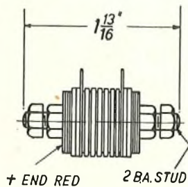
FIG. 1.—WESTINGHOUSE RECTIFIER.
