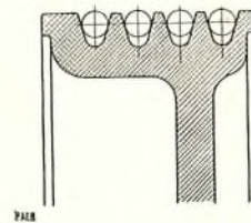
FIG. 5.—STANDARD VEE SHEAVE.
