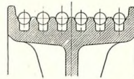
FIG. 4.—SPECIAL SHEAVE.
