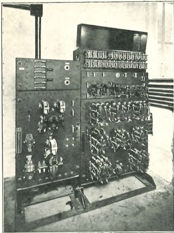
FIG. 9.—CONTROLLER.
