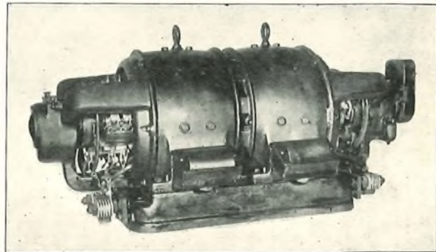
FIG. 8.—MOTOR-GENERATOR SET.
