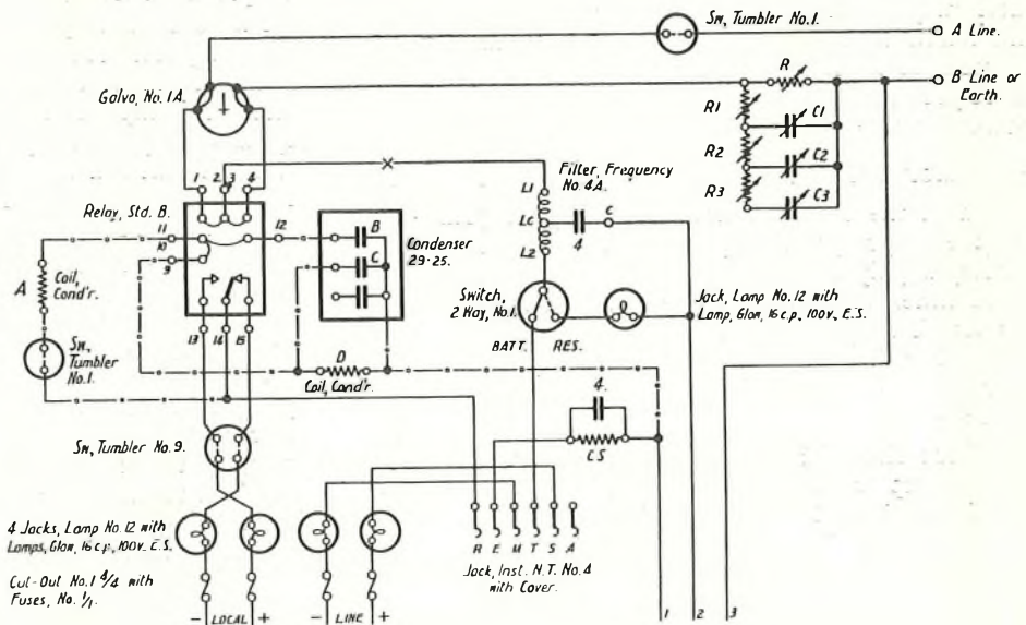
FIG. 2.—TELEPRINTER DUPLEX CIRCUIT.
