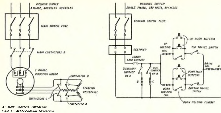
FIG. 2.—WIRING DIAGRAM.
