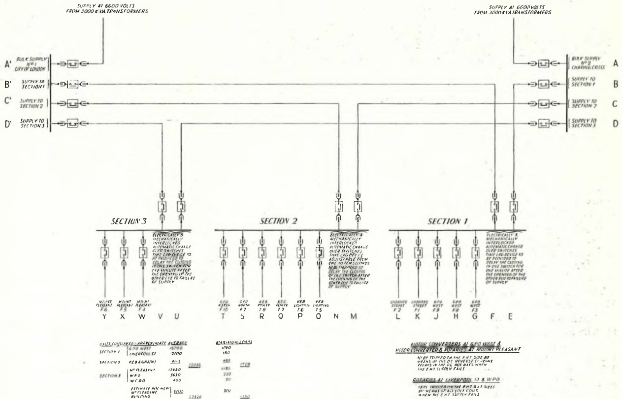
FIG. 4.—CONNEXIONS OF E.H.T. SWITCHGEAR.
