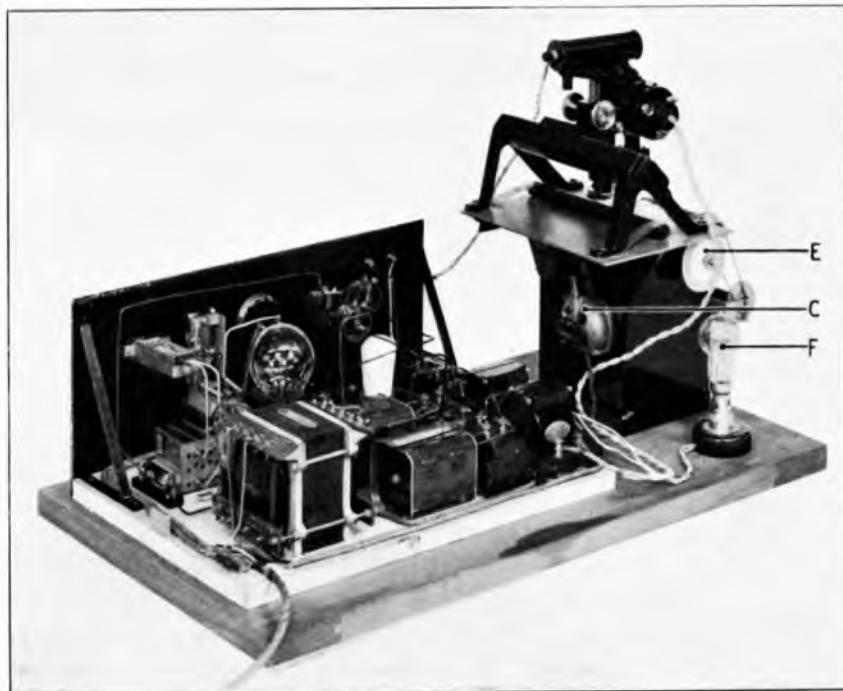
FIG. 2.—CHART ANALYSER.
