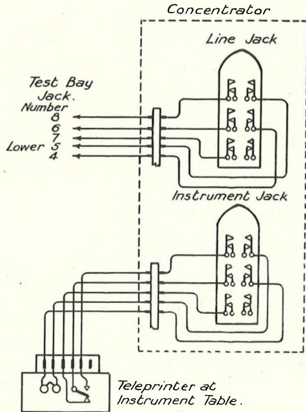
FIG. 7.—CONCENTRATOR CONNEXIONS.
