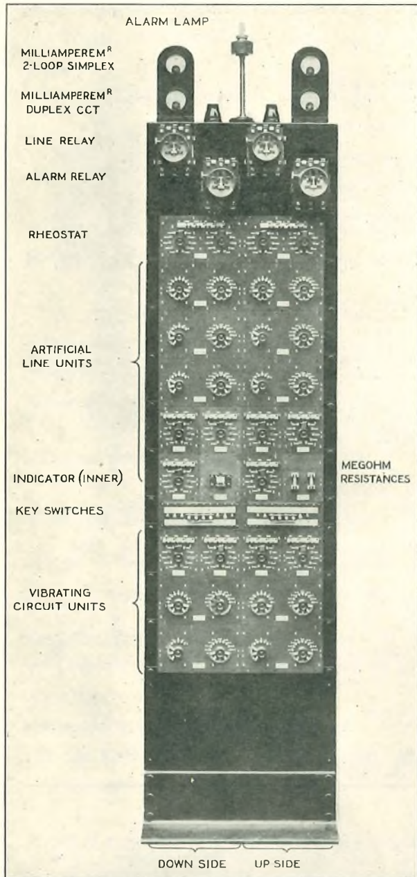
FIG. 4.—APPARATUS BAY.
