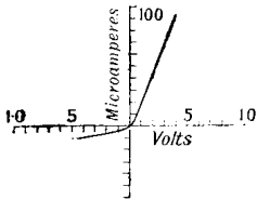
BORNITE-ZINCITE CURVE
