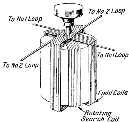
RADIOGONIOMETER CONNEXION
