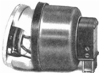
Fig. 44—S. T. & C. MICROPHONE 4017A
