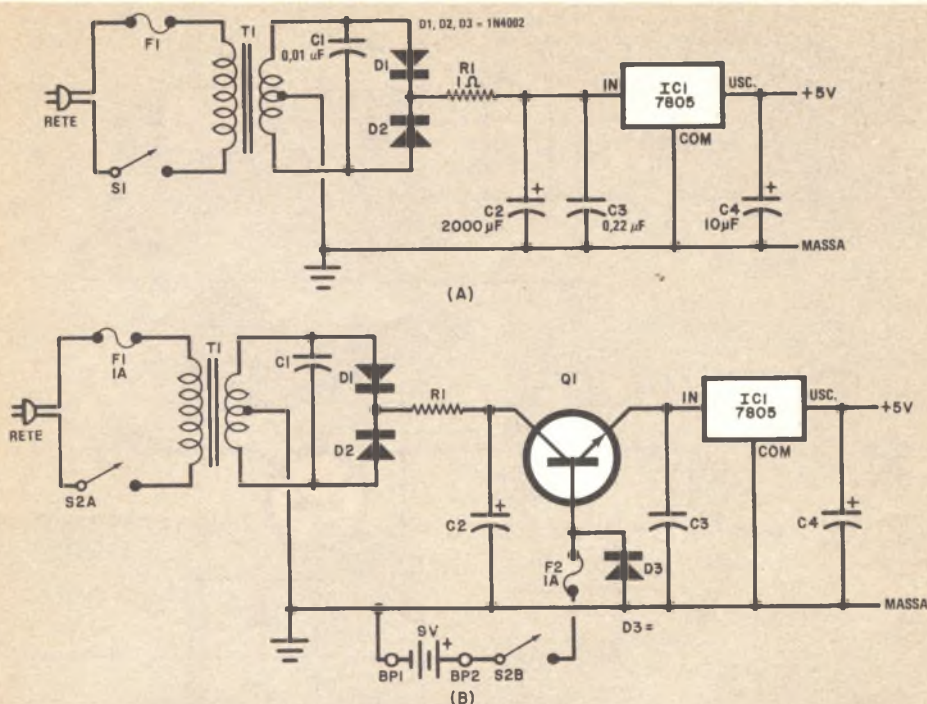
Fig. 3 - Circuito dell'alimentatore nella versione a sola rete (A); circuito previsto per il funzionamento dell'alimentatore con batteria di riserva (B).
