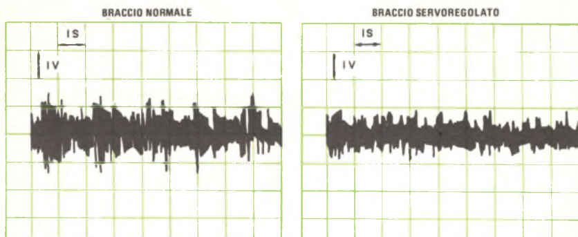
Fig. 3 - Un braccio stabile può ridurre decisamente, su un'estesa banda di frequenza, il rumore in uscita dalla testina.
