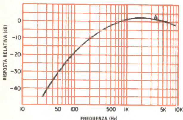
Fig. 5 - La curva di pesatura "A" (a lato) riflette l'andamento della sensibilità uditiva in funzione della frequenza, valutata in corrispondenza di un livello di ascolto di 70 phon. Il circuito mostrato in basso consente di ottenere la pesatura secondo la curva "A", adattando l'impedenza d'uscita di 600 \Omega all'elevata impedenza d'ingresso dello strumento di misura.
