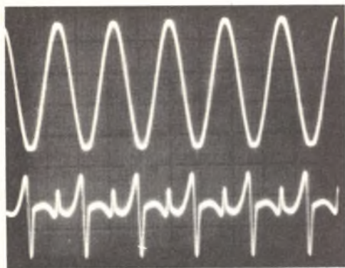
Fig. 6 - Il segnale d'uscita (rappresentato in alto), prodotto dall'amplificatore pilotato in zona di tosatura moderata delle creste del segnale, è affetto da una distorsione armonica totale dell'1%, secondo quanto è indicato da un analizzatore di distorsione, la cui uscita è illustrata nella traccia inferiore.
