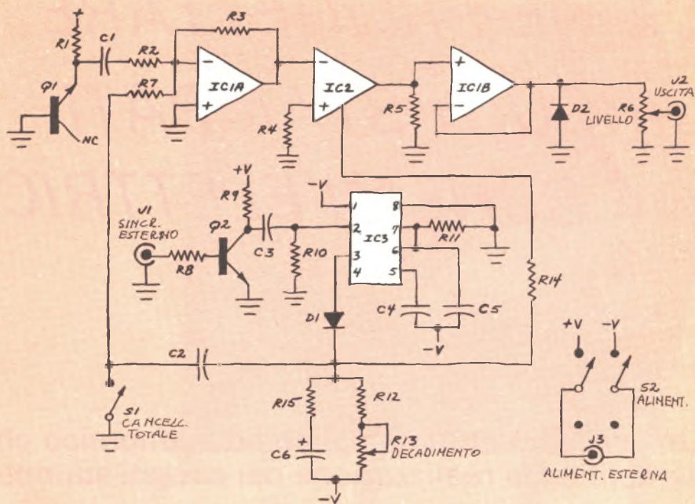
Fig. 1 - Esempio di circuito per il quale si vuole realizzare il circuito stampato. Si veda l'inserto "Come funziona" per quanto riguarda i dettagli circuitali.
