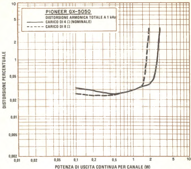
Distorsione armonica totale su 4 Ω e 8 Ω.
