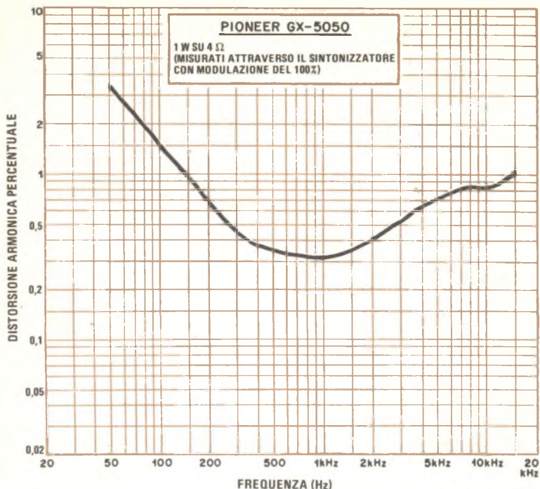
Distorsione armonica su 4 Ω.
