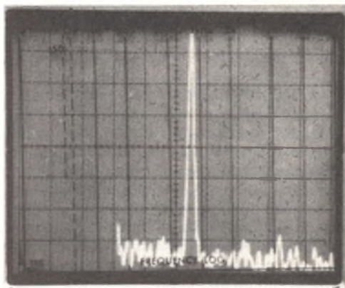
Fig. 9 - L'analisi spettrale dell'uscita a basso livello dell'amplificatore mostra che ogni prodotto di distorsione armonica è così basso da risultare mascherato dal tappeto di "erbetta" prodotto dal rumore.
