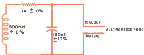
Fig. 4 - Schema elettrico del circuito da collegare agli ingressi fono per cartuccia a magnete mobile del preamplificatore per eseguire le misure di rumore.
