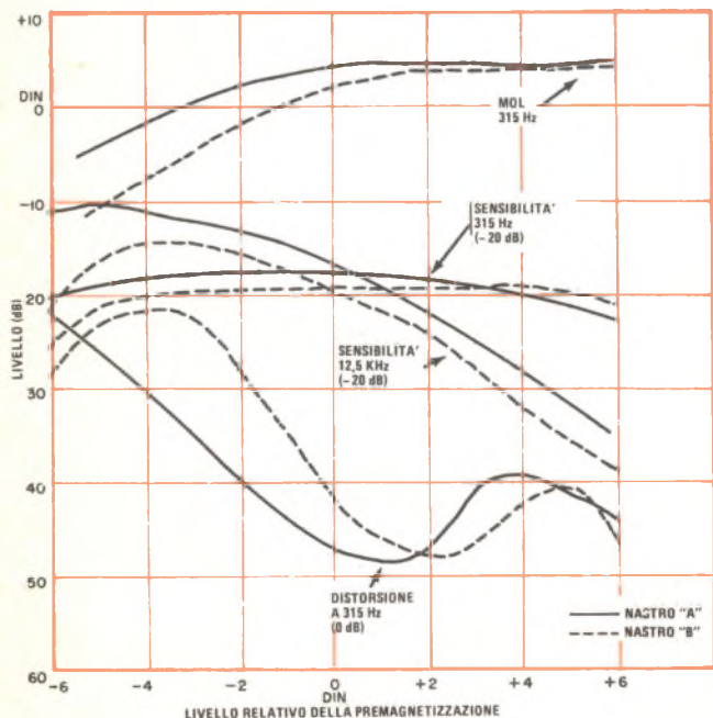
Fig. 1 - Le curve pongono a confronto le prestazioni di due diversi tipi di nastro (A e B) mettendo in evidenza gli effetti della premagnetizzazione.
