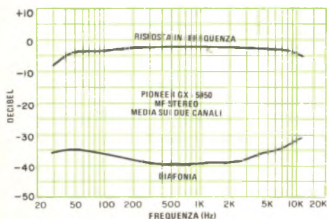
Risposta in frequenza e diafonia.
