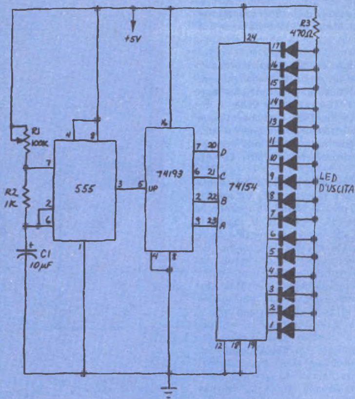
Fig. 7 - Circuito sequenziatore 1 di 16.
