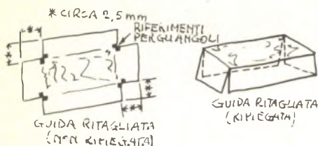
Fig. 4 - E' conveniente tagliare e ripiegare la guida definitiva come è illustrato in questa figura.
