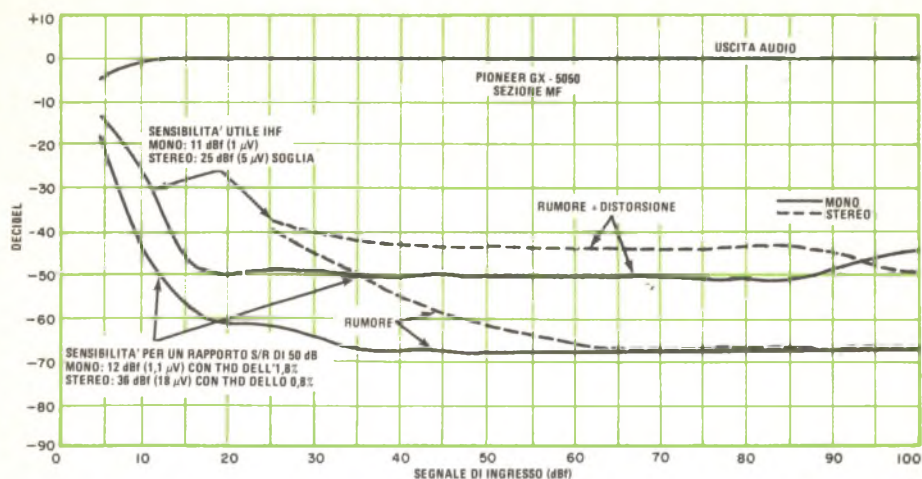
Curve di rumore e sensibilità per il Mod. GX-5050.
