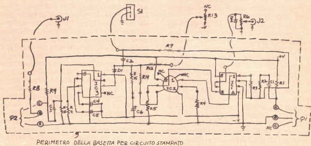
Fig. 2 - Si ridisegni il circuito secondo la disposizione fisica che i vari componenti assumeranno.
