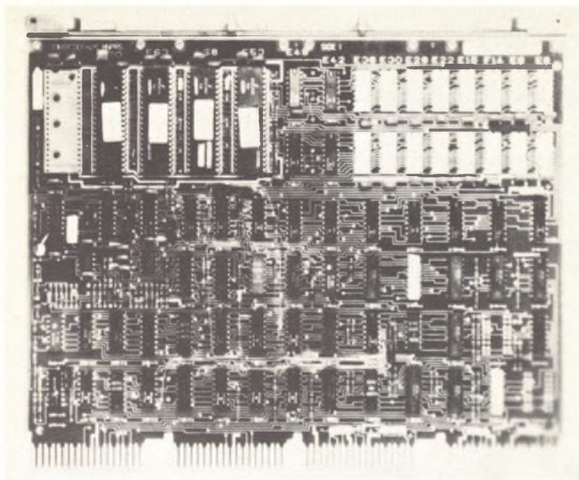
L'unità centrale di elaborazione usata nell'elaboratore H11, della Heath, rappresentata qui sopra, è molto più complessa di quella a 8 bit illustrata nella pagina accanto. Questa piastra contiene anche una RAM (memoria ad accesso casuale) da 4K; su entrambe le piastre sono installati i necessari circuiti integrati ausiliari.
