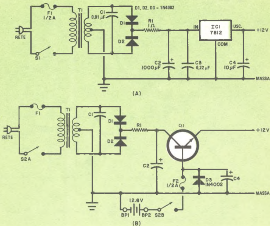
Fig. 4 - Alimentatore a rete (A) e circuito con batteria di riserva (B).
