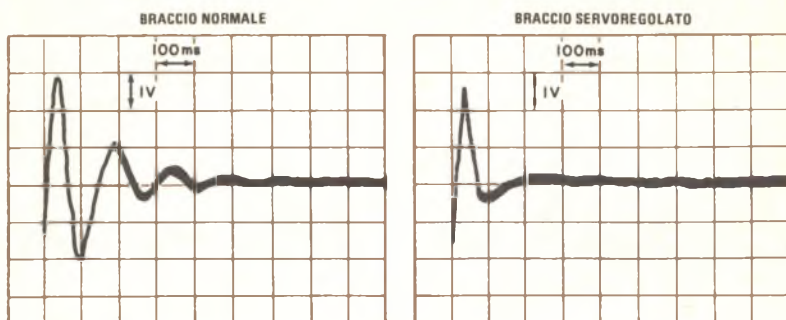
Fig. 4 - Da questa prova d'urto, la superiorità di un braccio servoregolato appare evidente dal rapido smorzarsi dell'oscillazione.
