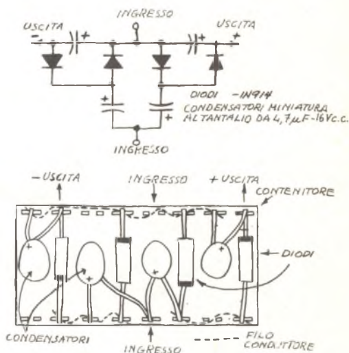
Fig. 2 - Schema elettrico e dettagli costruttivi di un moltiplicatore di tensione miniaturizzato a quattro stadi.
