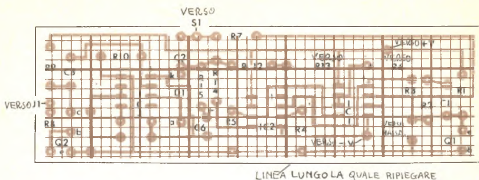
Fig. 3 - Ecco come si deve presentare un lavoro eseguito esattamente in scala. Risulta conveniente utilizzare carta millimetrata per poter collocare le piazzole con precisione.
