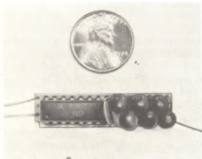
Fig. 4 - Prototipo montato del circuito della fig. 3.
