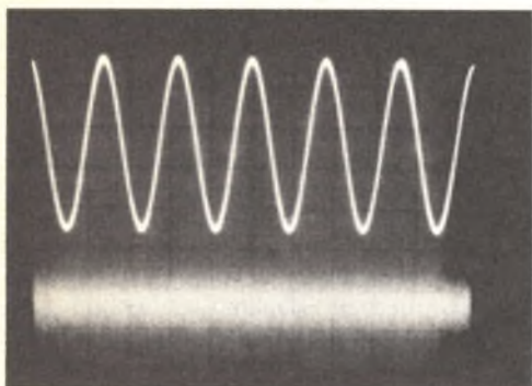
Fig. 8 - Quando la potenza d'uscita erogata dall'amplificatore viene ridotta a 0,25 W (traccia superiore), l'uscita dell'analizzatore di distorsione (traccia inferiore) consiste quasi interamente nel rumore.
