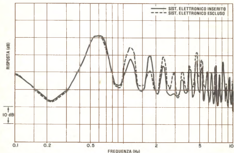
Fig. 1 - Prove eseguite sul braccio Sony con il sistema elettronico inserito (linea continua) ed escluso (linea a tratti) per mostrare gli effetti delle fluttuazioni lente e rapide di velocità ("wow" e "flutter") fino a 10 Hz.
