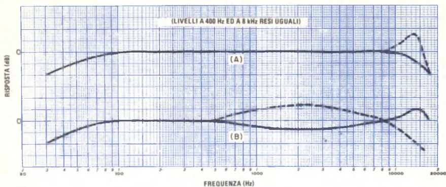
Fig. 2 - Possibili differenze tra le risposte di due diversi nastri. In a) sono visibili due risposte molto simili tra loro, ma in altri casi (b) la differenza può essere notevole.
