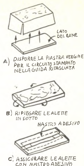
Fig. 5 - Sono qui illustrate le tre fasi del lavoro finale: in A) si ricopre la basetta vergine per circuito stampato con la guida ritagliata, in B) si ripiegano le alette in sotto, fissando poi il tutto con nastro adesivo (C).
