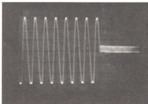
Fig. 3 - La porzione del segnale per la misura del margine dinamico della potenza d'uscita, costituita da un treno di oscillazioni, provoca l'erogazione di una potenza d'uscita superiore a quella nominale.
