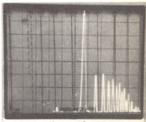
Fig. 7 - Analisi spettrale del segnale d'uscita, prodotto dall'amplificatore, mostrato nella traccia superiore della fig. 6.
