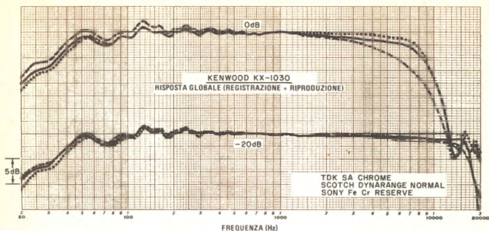
Risposta in frequenza misurata a due diversi livelli di registrazione e con tre tipi diversi di nastro.
