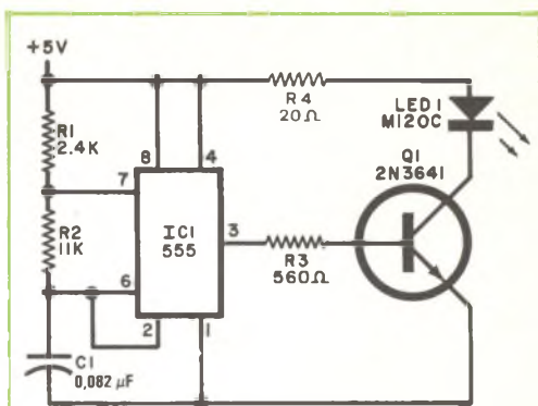
Fig. 1 - In questo semplice trasmettitore, il temporizzatore pilota Q1 per accendere il LED.
