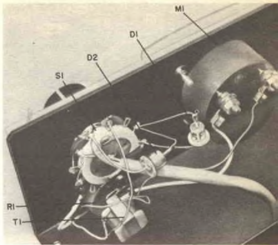
Fig. 2 - I componenti si montano direttamente sui terminali del commutatore, del potenziometro e dello strumento.
