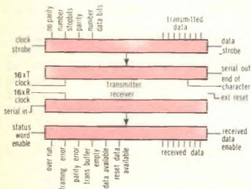
Fig. 4 - Schema del circuito MOS/LSI AY-5-1012 (UAR/T) della General Instrument Europe.
