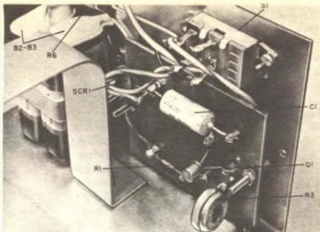
Il circuito stampato si fissa alla scatola mediante distanziatori da 10 mm. La staffetta a U a sinistra serve per B1.
