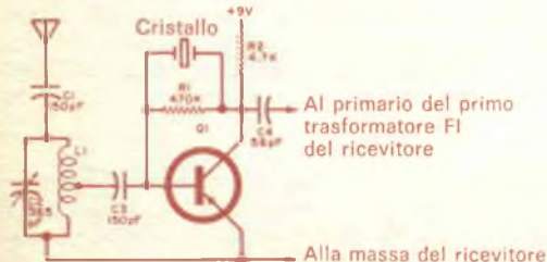
Ecco il circuito del convertitore progettato per l'uso con un radiorecettore portatile a transistori.
