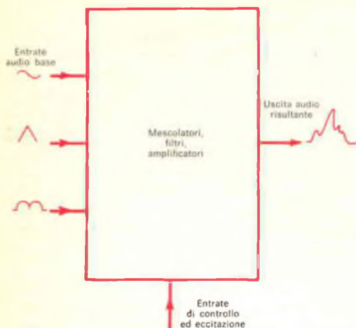
In questo schema base di un sintetizzatore, si vedono le entrate audio combinate in uscite complesse. L'operatore controlla l'uscita finale.
