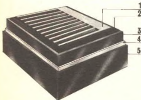
Fig. 1 - Struttura di una cella solare di tellururo di cadmio a film sottile: 1) elettrodo in oro, 2) tellururo di rame spesso da 200 Å a 300 Å 3) tellururo di cadmio spesso da 10 µm a 15 µm, 4) sulfuro di cadmio spesso 1 µm, 5) molibdeno spesso da 15 µm a 25 µm.
