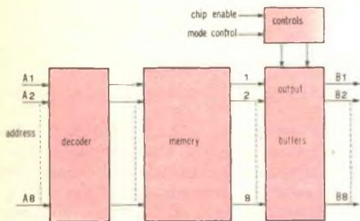
Fig. 3 - Schema della memoria a sola lettura RO-6-2048 della General Instrument Europe.
