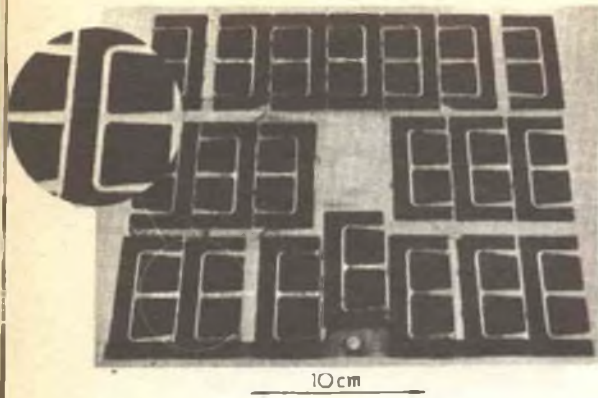
Fig. 2 - Fotografia di un modulo di cella solare al CdTe per l'alimentazione degli strumenti nei palloni-sonda degli atrimenti nei palloni-sonda meteorologici.
