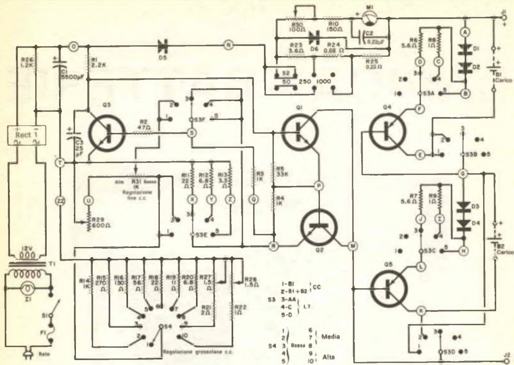
Fig 1 - Le lettere racchiuse nei cerchietti si riferiscono ai terminali del telaio perforato principale. Le posizioni indicate per S3 e S4 devono essere riportate in modo identico sul pannello frontale.
