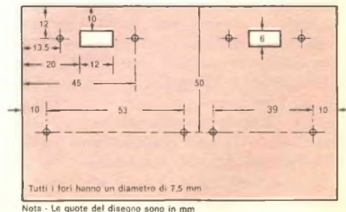
Fig. 2 - Piano di foratura del pannello anteriore della scatola. Se si usano commutatori a pallina, anziché fori rettangolari, si devono praticare fori rotondi.
