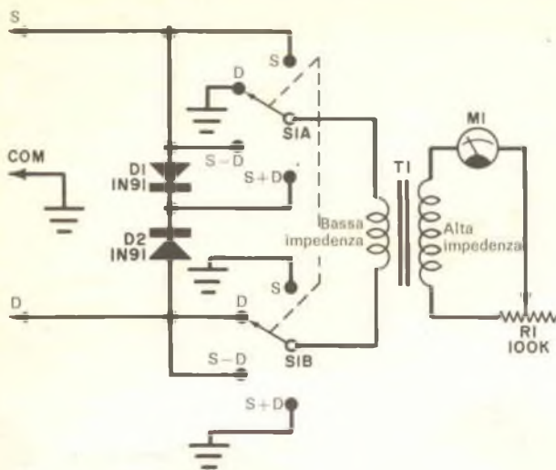
Fig. 1 - Il circuito del misuratore di bilanciamento consiste essenzialmente in un sistema in salita che pilota lo strumento. I diodi assicurano l'isolamento.
