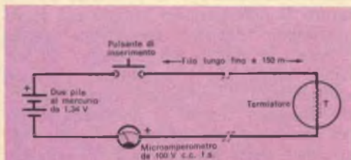
Fig. 1 - Ecco l'illustrazione del circuito base di un termometro elettrico impiegante un termistore EMC4; la gamma di funzionamento del dispositivo è compresa fra -17,8 °C e +45 °C.
