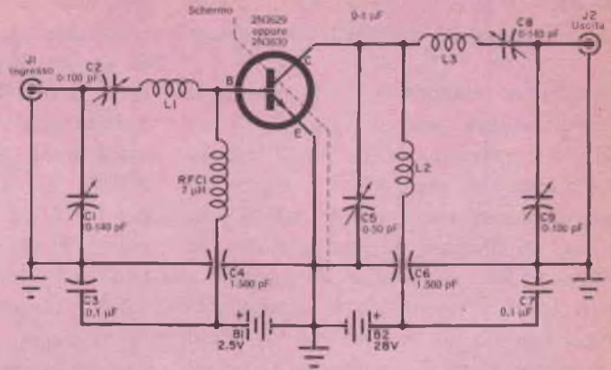
Fig. 1 - Questo amplificatore di potenza a 15 W 50 MHz è stato progettato per l'uso di transistori al silicio della serie che comprende i tipi 2N3627, 2N3628, 2N3629, 2N3630. Il progetto base può essere modificato per applicazioni con frequenze diverse e differenti livelli di potenza.
