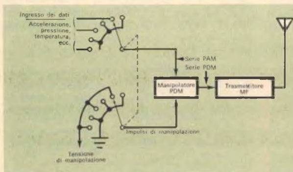
Fig. 5 - Ad ogni dato di ingresso proveniente da ciascun trasduttore viene assegnato un contatto del commutatore. A mano a mano che l'accelerazione, la pressione o la temperatura vengono sentite, il contatto rotante del commutatore preleva le tensioni corrispondenti e le applica all'entrata del manipolatore. Questo converte gli impulsi di ampiezza variabile (PAM) in impulsi di larghezza variabile (PDM) i quali possono modulare in frequenza il trasmettitore.
