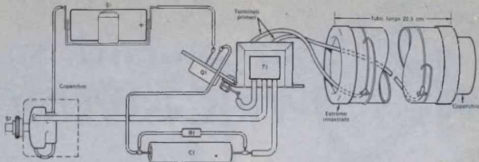
Tutti i componenti, compresa la batteria, trovano posto nel tubo di cartone. I terminali provenienti dall'avvolgimento primario di T1 fuoriescono dal tubo e sono ricoperti da strisce di alluminio. Gli elettrodi, larghi circa 10 cm, sono distanziati fra di loro di circa 2,5 cm.
