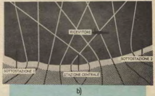
Fig. 2 - Le figure indicano i due sistemi in cui Hi-Fix può essere impiegato. Nel sistema a due campi (a) vi sono due sottostazioni a riva e la stazione centrale sull'imbarcazione insieme al ricevitore: questa soluzione offre la massima precisione ottenibile, con solo due stazioni sulla costa e carta senza reticolo. Nel sistema iperbolico (b) le due sottostazioni e la stazione centrale sono sulla costa ed il ricevitore, da solo, sulla nave. Questo sistema offre un servizio assai preciso contemporaneamente ad un numero illimitato di utilizzatori, ciascuno dei quali necessita solo di un suo piccolo ricevitore.
