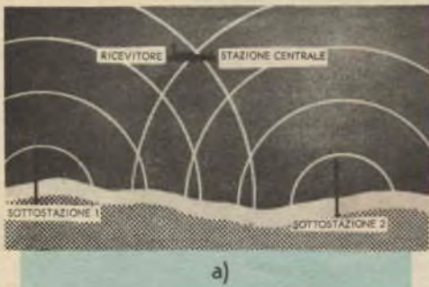
Fig. 2 - Le figure indicano i due sistemi in cui Hi-Fix può essere impiegato. Nel sistema a due campi (a) vi sono due sottostazioni a riva e la stazione centrale sull'imbarcazione insieme al ricevitore: questa soluzione offre la massima precisione ottenibile, con solo due stazioni sulla costa e carta senza reticolo. Nel sistema iperbolico (b) le due sottostazioni e la stazione centrale sono sulla costa ed il ricevitore, da solo, sulla nave. Questo sistema offre un servizio assai preciso contemporaneamente ad un numero illimitato di utilizzatori, ciascuno dei quali necessita solo di un suo piccolo ricevitore.
