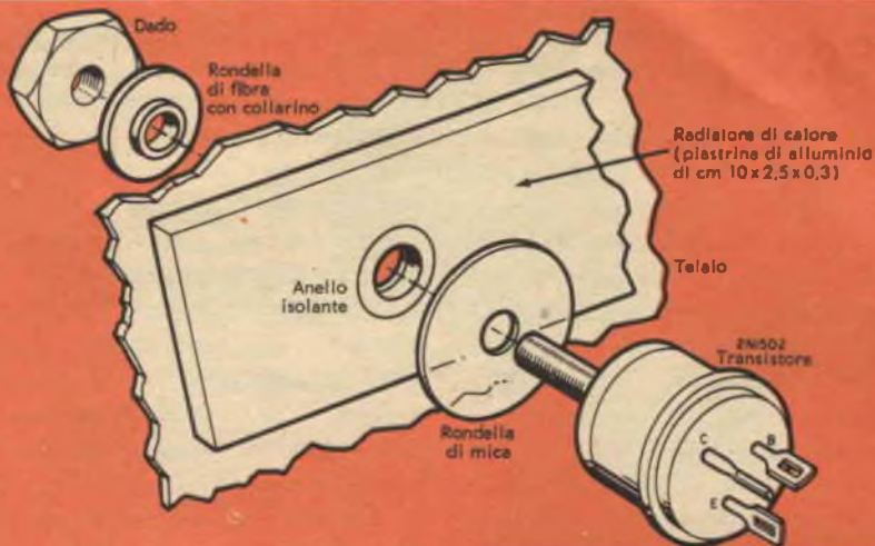
Fig. 2 - Nel montaggio dei transistori si usa un radiatore di calore per disperdere il calore ed anche per isolare i transistori dal telaio.
