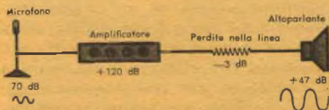
Fig. 3 - Il livello del microfono di -70 dB viene portato al livello di +47 dB dell'altoparlante dall'amplificatore che ha un guadagno di +120 dB.
