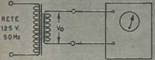
TESTER PER C.A. 10V FONDO SCA. LA 1000 Ω/V
