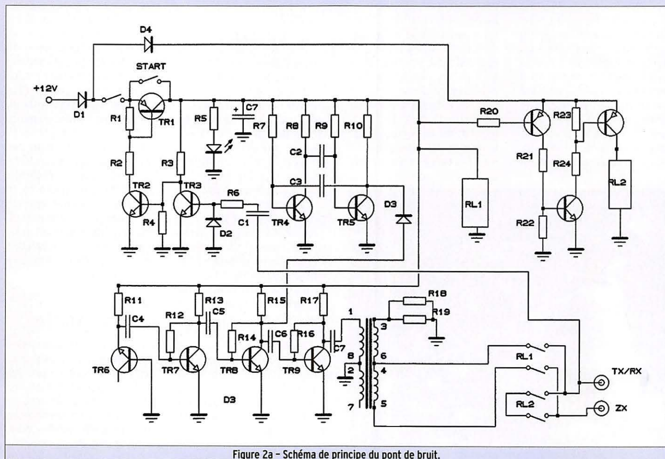
Figure 2a - Schéma de principe du pont de bruit.
