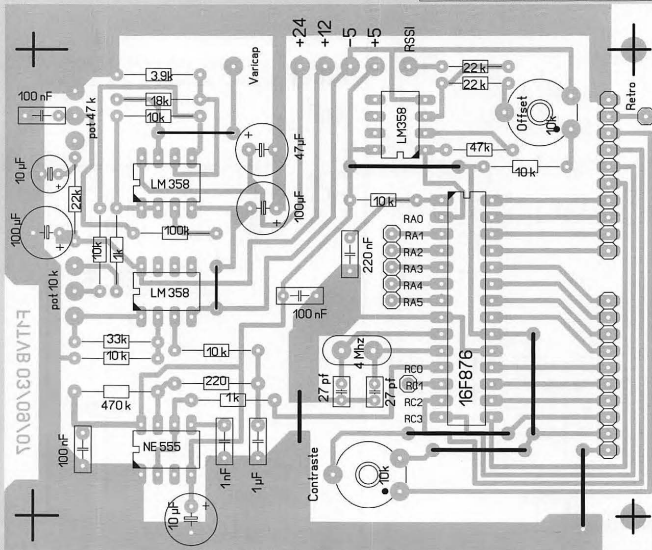
7 - Implantation des composant de la carte PIC.
