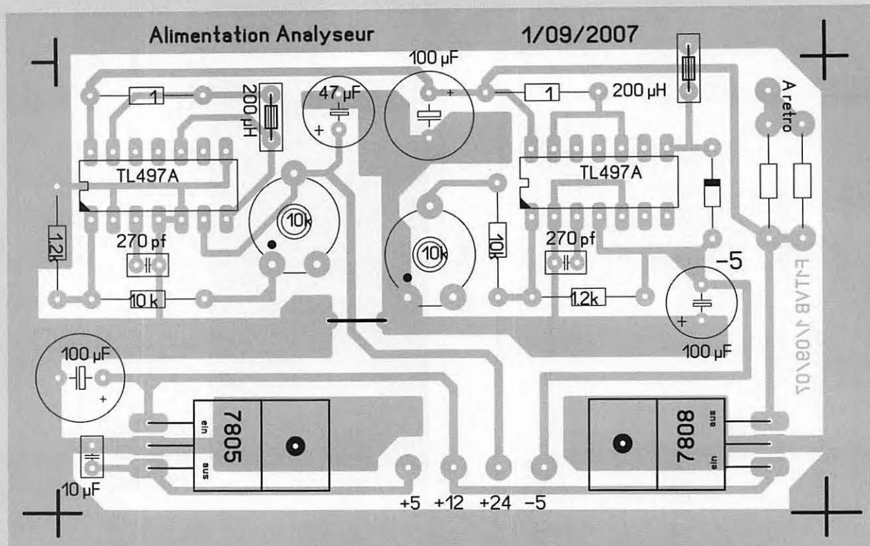
6 - Implantation des composants de la carte alimentation.
