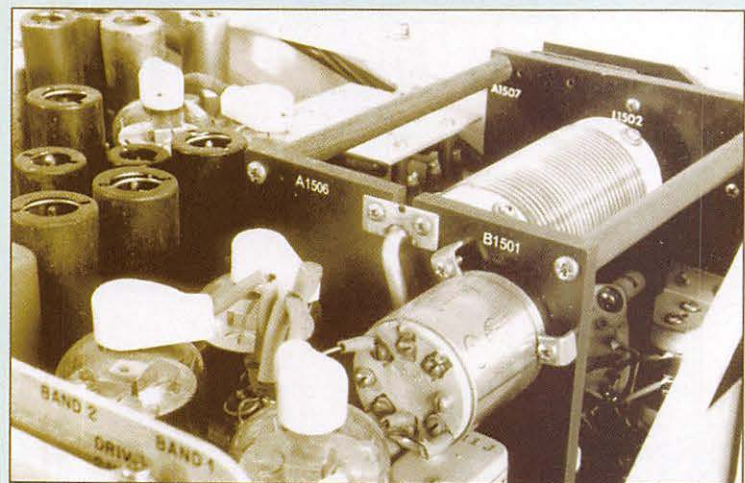
7 - Au premier plan le PA, au fond les 2 tubes du modulateur.
