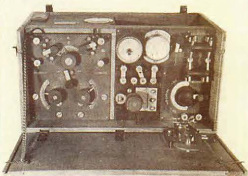
4 - Poste E/R type E3 (1re Guerre Mondiale).
