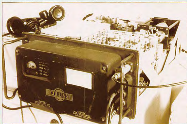
1 - Le 618S-1 vu de face, capot enlevé.
