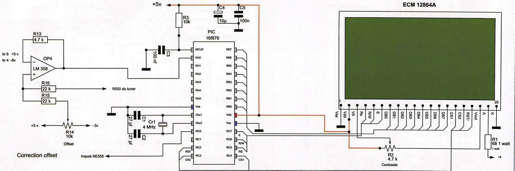
Générateur de rampe pour analyseur -Tuner et correcteur offset RSSI - PIC 16F876 et LCD graphique
