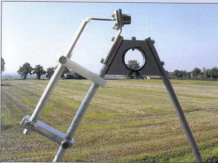
5 - Détail du gamma-match.
