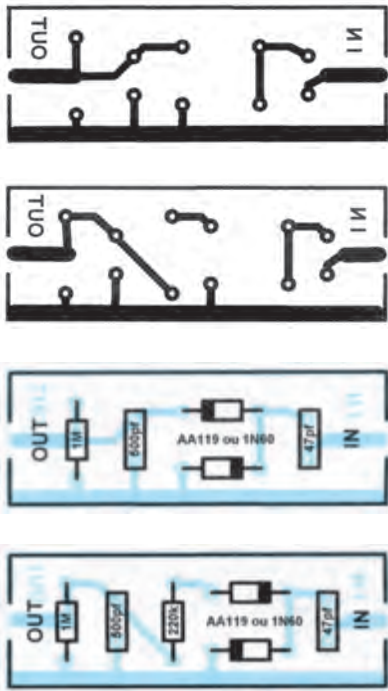
15a Pour l'alignement du transformateur discriminateur FM, ce réglage n'est pas plus compliqué qu'autre chose, il suffit pour cela de respecter la méthode. En se reportant au dessin (figure 12) qui représente 15b 16a 16b
