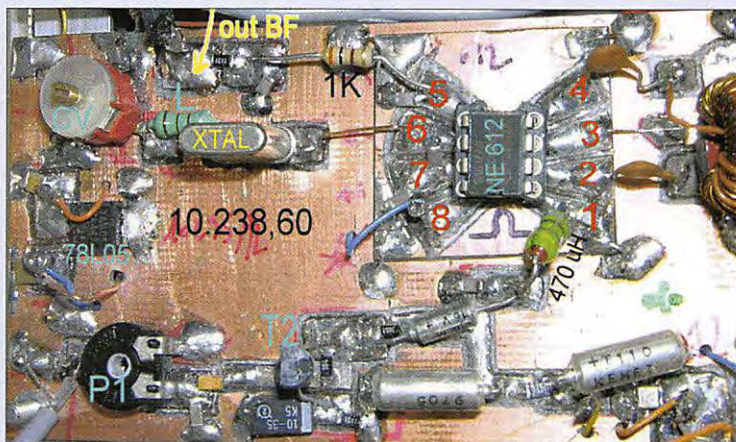
Photo 13 – Générateur DSB détecteur de produit.
