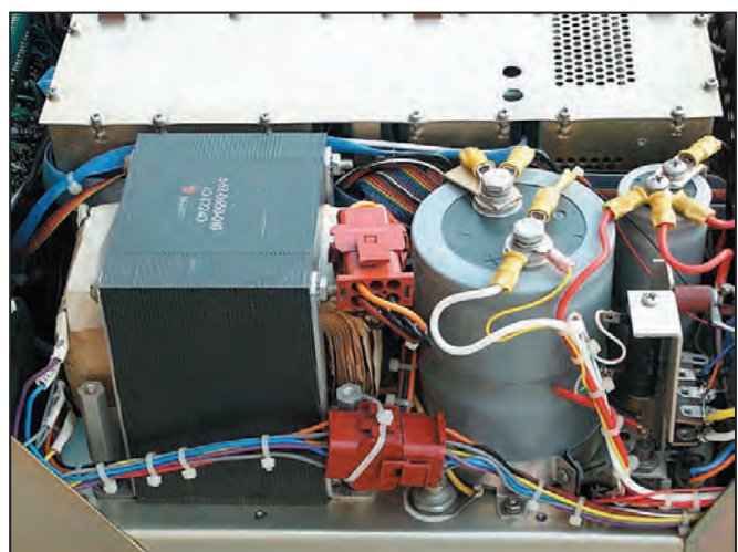
6 - Alimentation interne.
