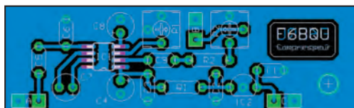
7 - Implantation des composants du compresseur.
