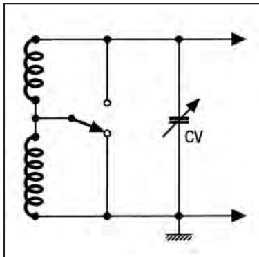
4 - Si on doit commuter entre plusieurs enroulements d'antenne, on a avantage à procéder par court-circuit du ou des enroulements non utilisés.
