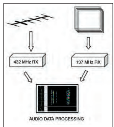
6 - Synoptique du système de réception.
