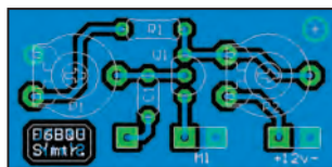
10 - Implantation des composants.
