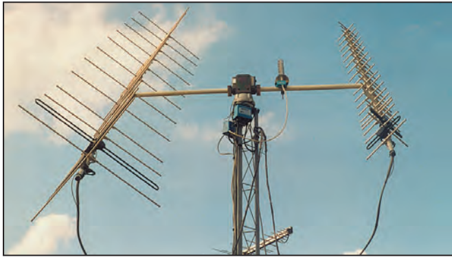
7 - Antenne de réception 144 MHz (à droite).
