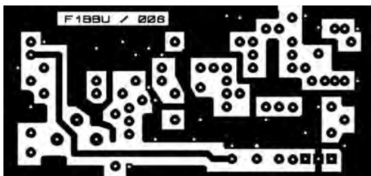
1B - CI platine VFO, côté composants.
