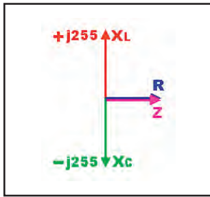
3 – Quand X_L et X_C s'annulent, Z est purement résistive.
