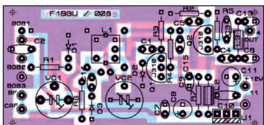
2C - Implantation des composants platine VFO.
