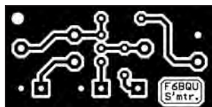
9 - Platine CI du S-mètre.
