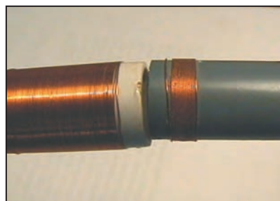
Figure 2: Bobines fortement couplées
