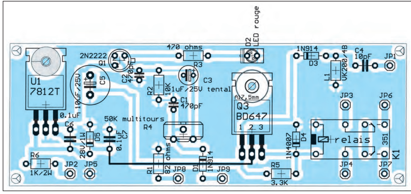
Figure 6 : Implantation des fonctions annexes.
