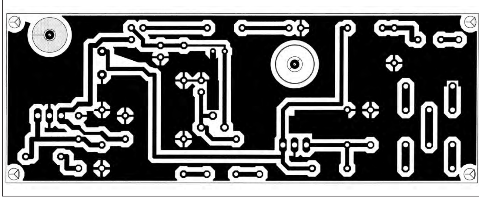
Figure 6 : Circuit imprimé des fonctions annexes.
