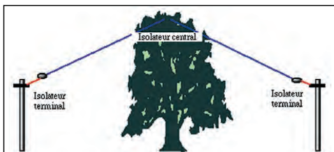
Figure L02 - Une Lévy en "V" inversé (version écologique).
