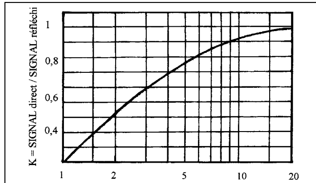
Figure 8 : ROS Rapport d'Ondes Stationnaires (tension ou courant).
