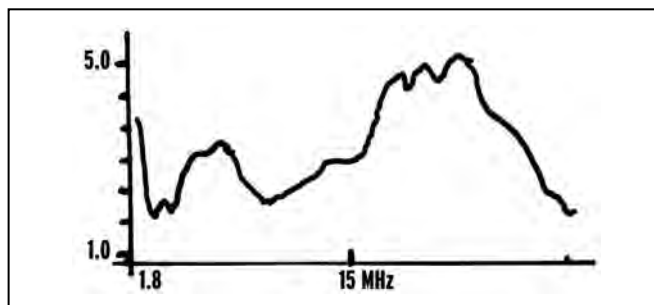
Courbe du ROS, sans coupleur, à 3 m, entre 1,8 et 30 MHz.
