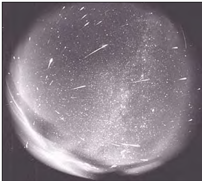
Essaim des Léonides vu par satellite.
