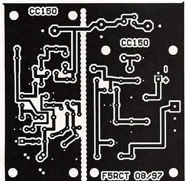
Circuit imprimé côté soudures.
