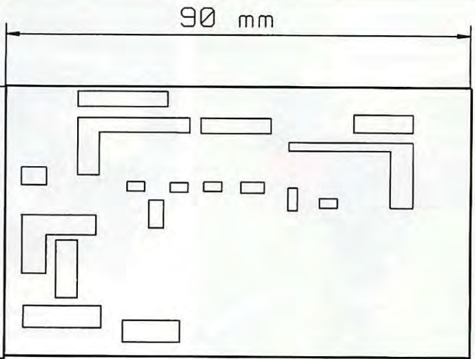
Plaque cuivrée époxy double face. - Laisser la face inférieure cuivrée. - A l'aide d'un cutter, isoler les zones indiquées côté composants.
