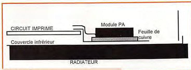
Figure 1 Montage du module hybride.
