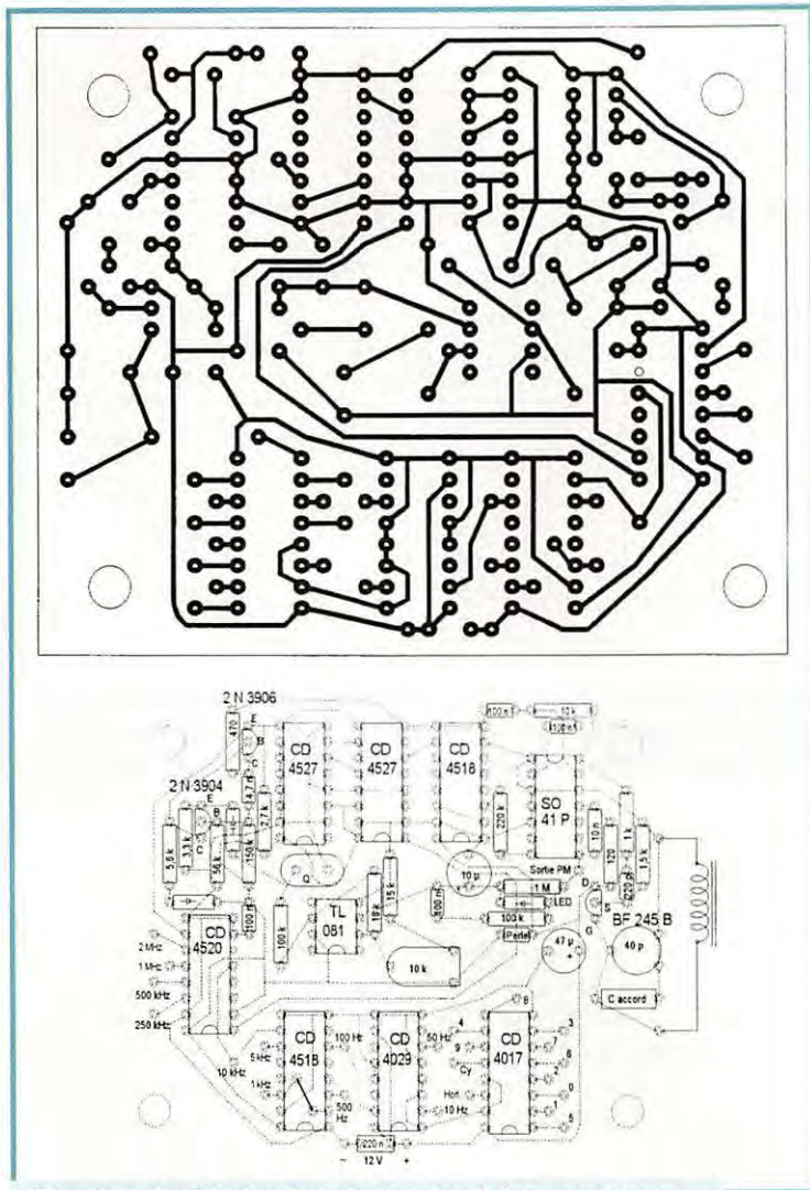
Fig. 4. — La platine imprimée réunit les montages des figures 3 et 4. Il convient de la blinder, pour éviter tout rayonnement sur le bâtonnet de ferrite.
