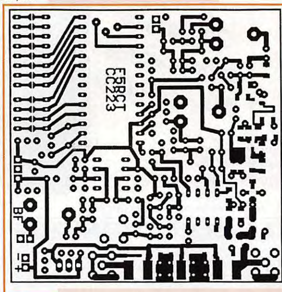
Cuivre côté composants.
