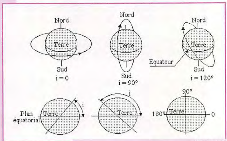
Figure 1 : Convention de la définition de l'inclinaison.
