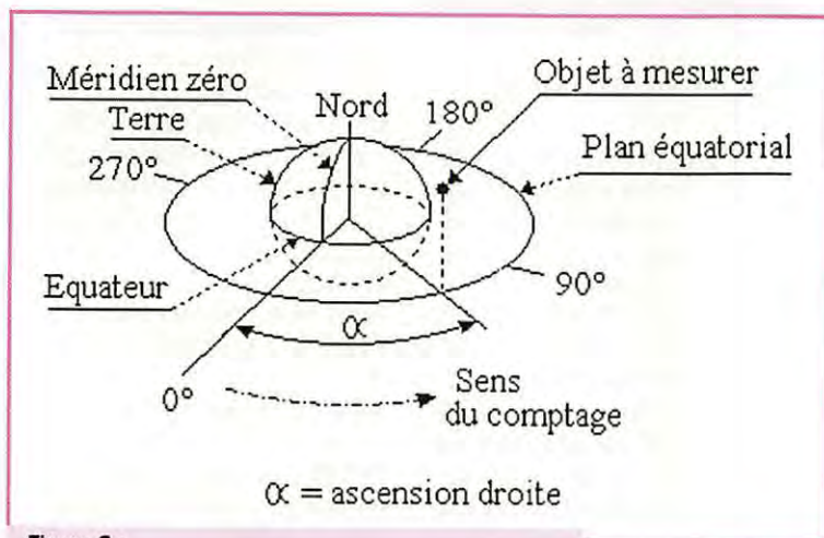
Figure 2 : Définition de l'ascension droite.
