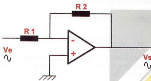
Figure 1 : amplificateur inverseur
