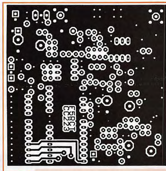
Cuivre côté soudures.
