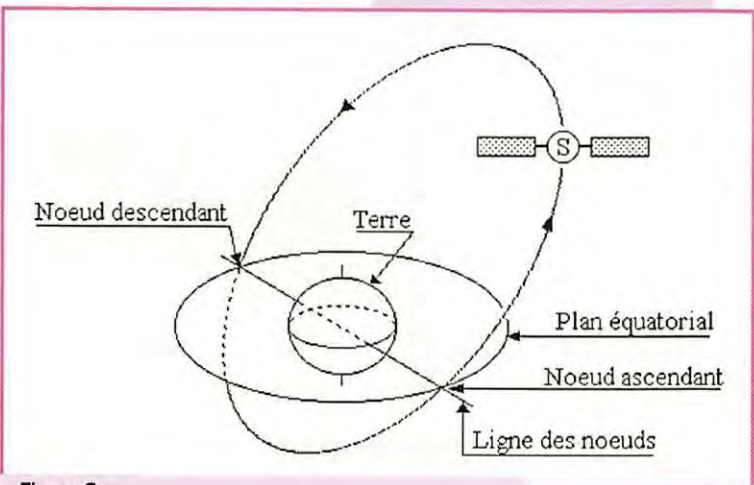
Figure 3 : Convention du nœud ascendant.
