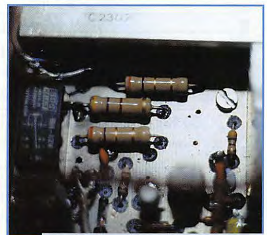
Détail de l'atténuateur.
