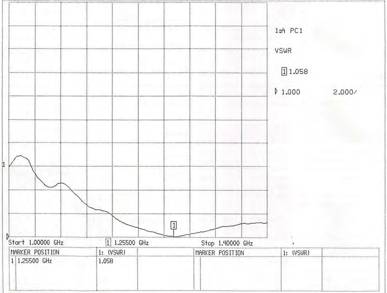
Courbe de RDS de l'antenne photographiée : 1.06 à 1255 MHz et 1.26 à 1280 MHz.
