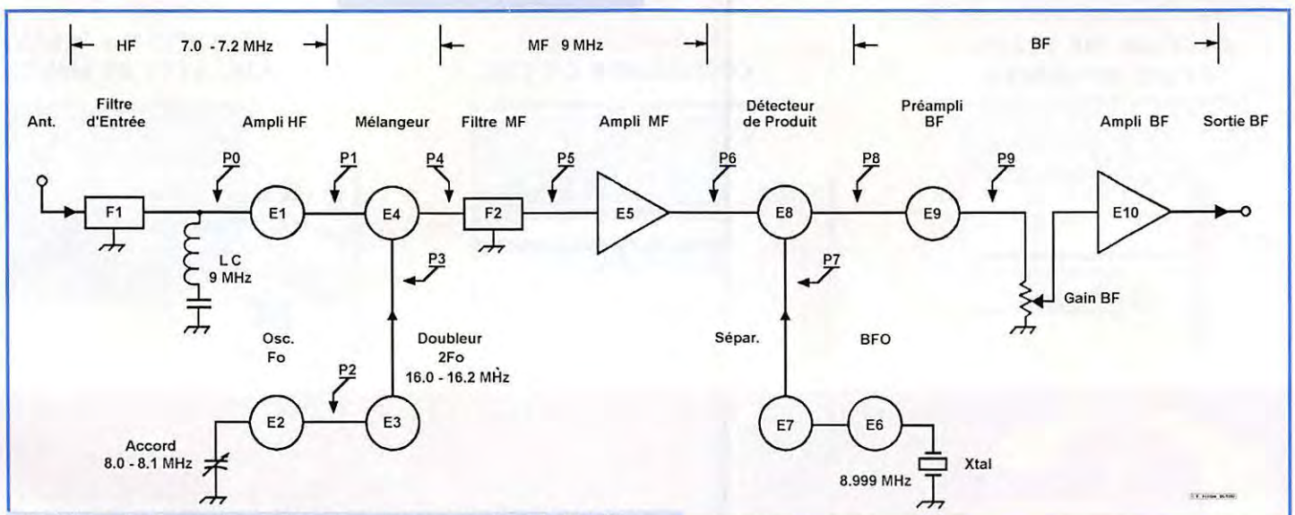
Schéma 1 : Synoptique d'un récepteur monobande 7 MHz, CW à simple changement de fréquence.
