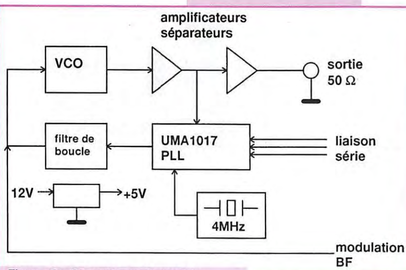
Figure 1 : Synoptique du module Synthétiseur.
