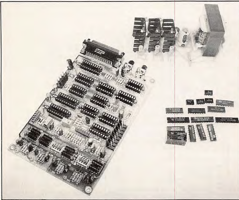
La carte principale et l'alimentation.
