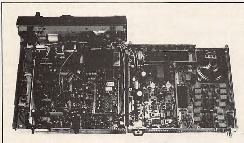
TS-680S chassis supérieur ouvert. De gauche à droite : le filtre CW en option, la carte "signal", l'étage final et les filtres passe-bas, à gauche desquels on distingue le circuit hybride 50 MHz.
