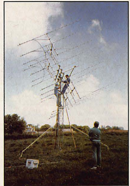
Montage des antennes.
