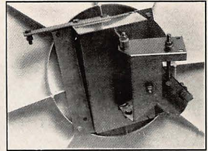
Photo 1 : Détail d'assemblage de la monture polaire.
