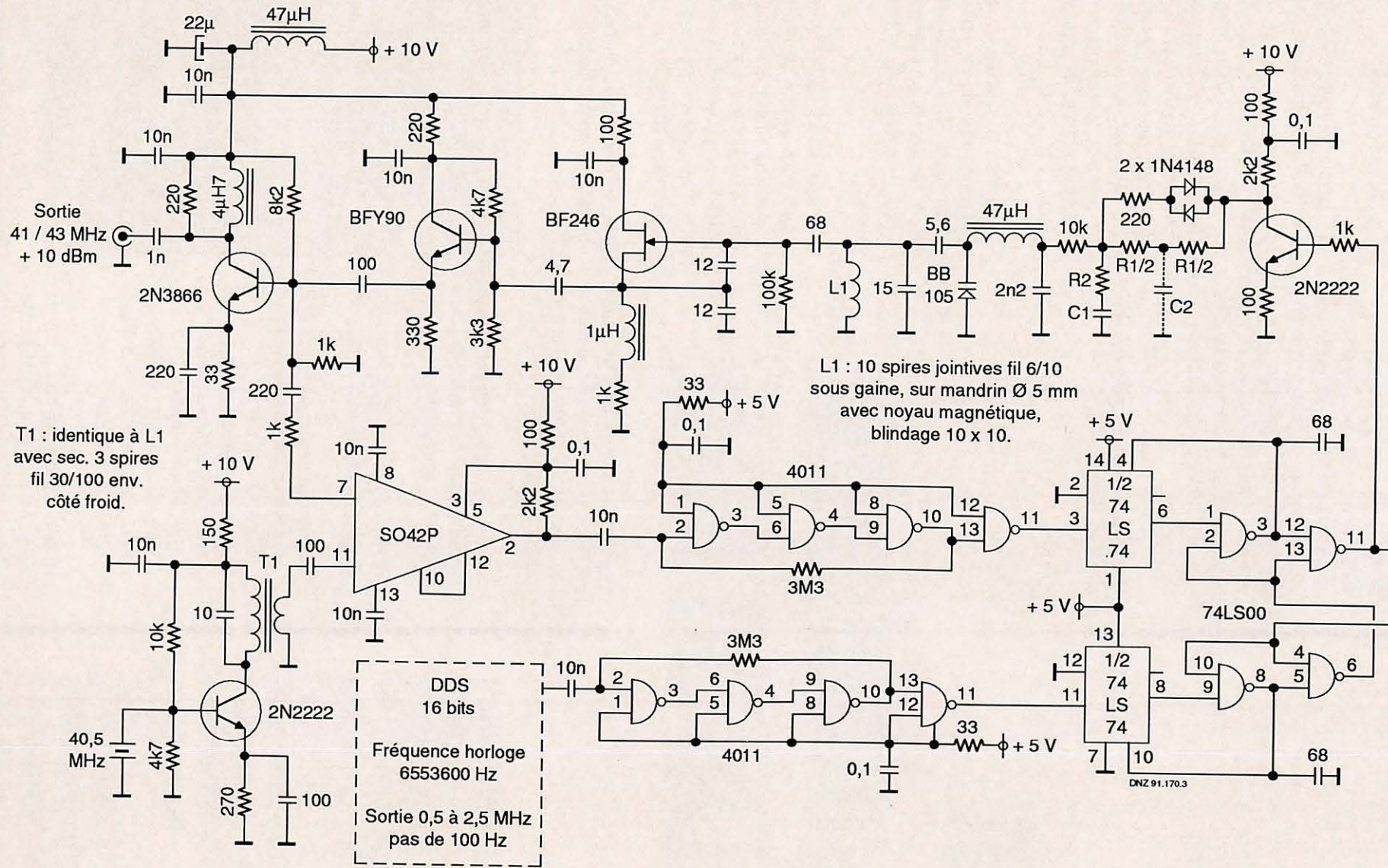
Figure 1 : Synthésiseur piloté DDS, prévu pour la bande 50 / 52 MHz avec FI 9 MHz.
