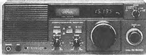
Récepteur R600. Prix : 3500 F Couverture générale 200 kHz à 30 MHz.
