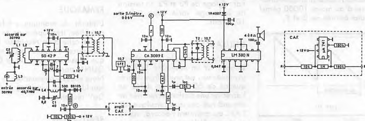
Figure 12 : L1 Ø 6 mm avec noyau 13 spires jointives sous fil plastique Ø4/10 mm. L2 Ø 6 mm avec noyau 3 spires jointives fil sous plastique Ø4/10 enroulé sur L1. L3 Ø 6 mm avec noyau 2 spires jointives fil sous plastique Ø4/10 enroulé sur L1. L4 Ø 6 mm avec noyau 7 spires jointives fil émaillé 4/10 enroulé sur H= 10 mm (H= hauteur bobine).
