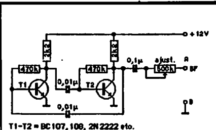
Balise 1000 Hz : l'ajustable de 500 k sert à régler le niveau d'injection de la BF qui ne doit pas être écarté dans le filtre 10,7 MHz céramique du récepteur
