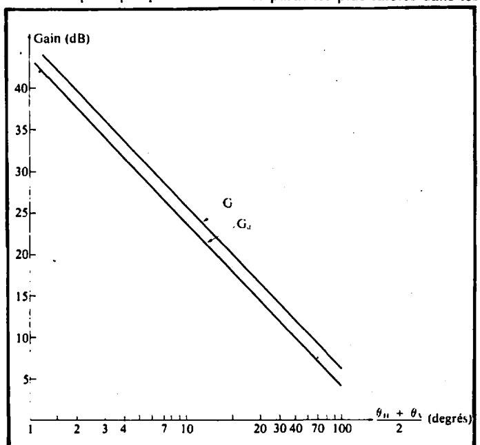
Fig. C.1.2c Courbes estimant le gain d'une antenne directive par rapport à la source isotrope et par rapport au doublet demi-onde en fonction de la moyenne \frac{\theta_H + \theta_V}{2} .
