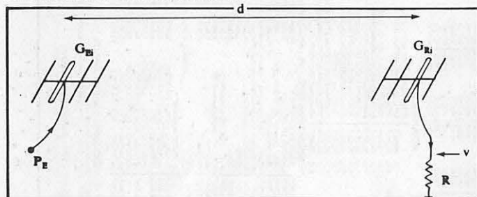
Fig. C.2.2c La tension v aux bornes de la résistance R est donnée par la formule v = \frac{\lambda}{4\pi d} \sqrt{P_E \cdot G_{Ei} \cdot G_{Ri} \cdot R} .
