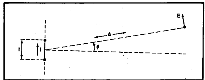
Fig. C.2.1a Le courant I crée à distance un champ électromagnétique dont la partie électrique est donnée par la formule E = \frac{60 \cdot \pi \cdot I \cdot l \cdot \cos \theta}{\lambda \cdot d \cdot \sqrt{2}} .
