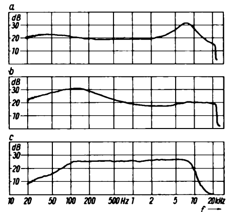
Bild 5. Frequenzkurven des kombinierten Aufnahme-Wiedergabe-Verstärkers; a = Aufnahme-frequenzgang, b = Wiedergabefrequenzgang, c = Frequenzgang über Band
