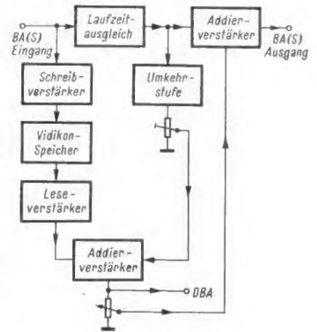
Bild 3. Blockschaltbild des vollständigen Geräts zur Aperturkorrektur. DBA = Differenzbild
