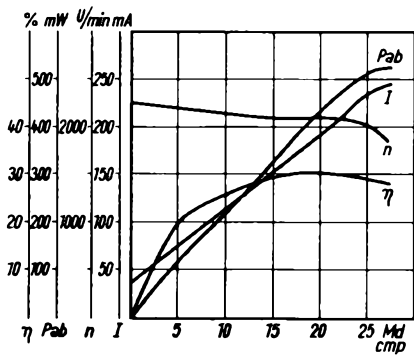
Bild 3. Die Drehmomentkennlinien des dreipoligen Gleichstrommotors, der im Optocord 450 verwendet wird
