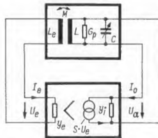
Bild 1. Funktionersatzschaltbild zur Ableitung der Rückkopplungsbedingung
