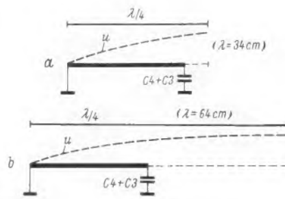
Bild 116. In UHF-Tunern mit \lambda/4 -Topfkreisen tritt der Spannungsknoten immer an derselben Stelle des Innenleiters auf, nämlich an dem mit Masse kurzgeschlossenen Ende. Die Spannungsverteilung a) gilt für die höchste und b) für die niedrigste Frequenz
