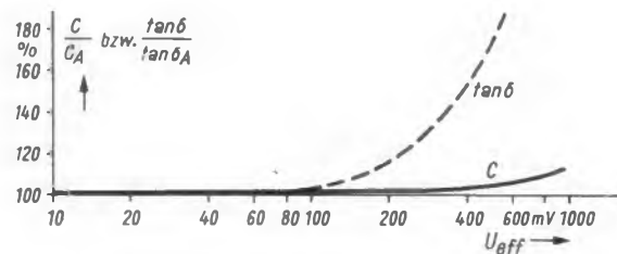
Bild 6. Wechselspannungsabhängigkeit der Kapazität und des Verlustfaktors bei der Meßfrequenz von 1 kHz
