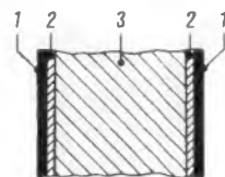
Bild 1. Querschnitt eines Sperrschichtkondensators; 1 = Silberbeläge, 2 = Sperrschichten des Keramikgrundkörpers, 3 = halbleitender Keramikgrundkörper
