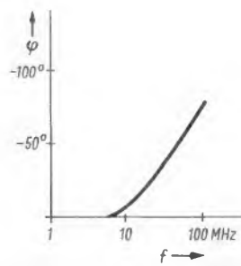
Bild 3. Verlauf des Phasenwinkels der Steilheit in Abhängigkeit von der Frequenz
