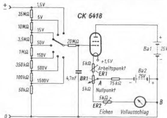
Bild 2. Prinzipschaltung für Gleichspannungsmessungen
