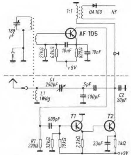
Bild 2. Weitere Empfangsleistungssteigerung durch zwei zusätzliche Transistoren T 1 und T 2. Die zusätzlichen Bauelemente sind unter die Trennlinie gezeichnet
