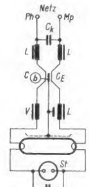
Bild 4. Hochwertige Entstörung einer Leuchtstofflampe in induktiver Schaltung L = Entstördrossel, C_E = Entstörkondensator mit Berührungsschutz C_b
