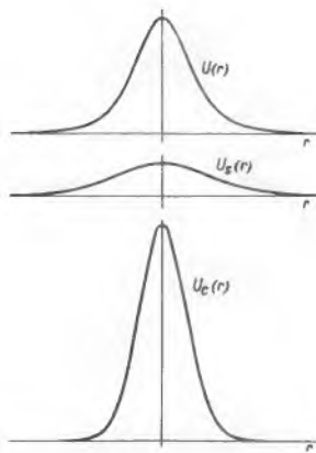
Bild 1. Schematische Darstellung der Aperturreinigung durch ein unscharfes Bild. Das aus dem zu korrigierenden Bildsignal hergestellt wird. U(r) ist die Abtastapertur der Kameraröhre, U_s(r) die des Speicherbildes und U_c(r) die korrigierte und verstärkte Apertur
