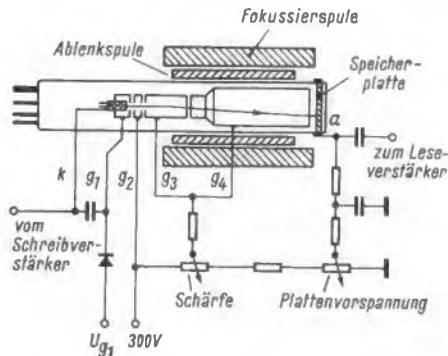
Bild 2. Betriebsweise des Vidikons als Signal-speicherröhre. Die Anschlüsse des Vidikons sind: k = Strahlkatode, g_1 = Wehneltzylinder, g_2 = Beschleunigungselektrode, g_3 und g_4 = Fokussierelektroden, a = Signalplatte. Die Speicherschicht wird zeitlich und örtlich konstant beleuchtet
