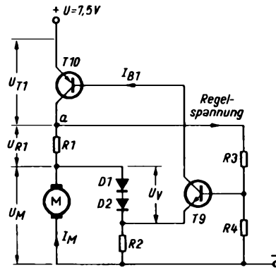
Bild 4. Prinzipschaltbild der Drehzahlregelung des Antriebsmotors
