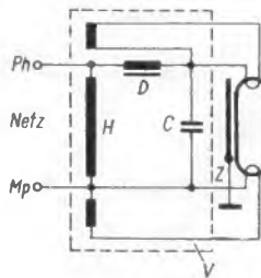
Rechts: Bild 2. Entstören einer starterlosen Leuchtstofflampe: H = Heiztransformator, Z = kapazitive Zündhilfe
