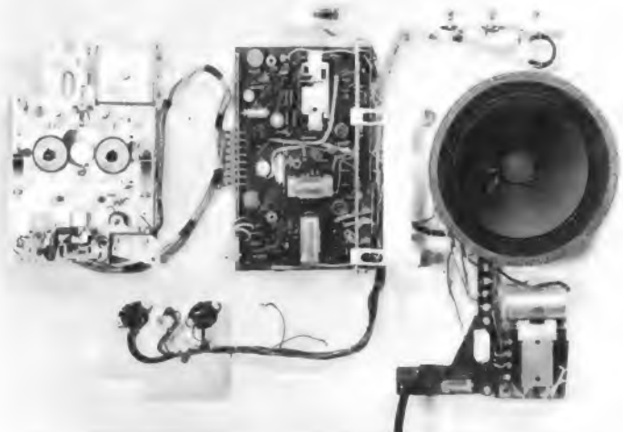
Bild 2b. Ansicht der demontierten Baugruppen des Kassetten-Tonbandgerätes. Die Verbindungsleitungen sind z. T. steckbar
