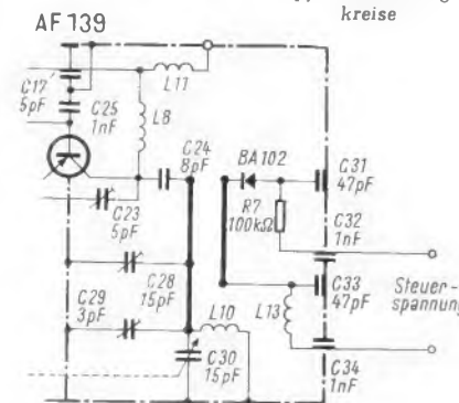
Bild 118. Schaltungsausschnitt eines UHF-Tuners mit einer Kapazitätsdiode für die automatische Oszillatornachstimmung (AFC)
