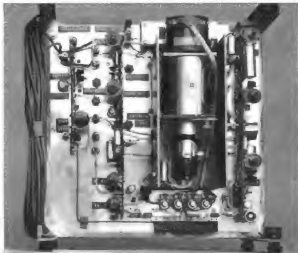
Bild 4. Das vollständig mit Transistoren bestückte Gerät zur Aperturkorrektur entsprechend der Blockschaltung in Bild 3
