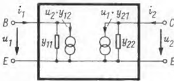
Bild 4. Vierpol-Parallelersatzschaltung für die Emitterschaltung
