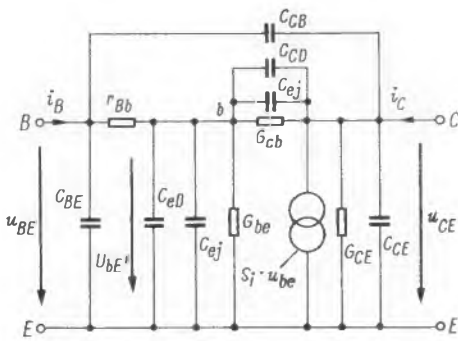
Bild 2. Ersatzschaltung für den Transistor in Emitterschaltung nach Giacoleto
