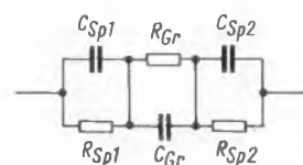
Bild 2. Ersatzschaltbild eines Sperrschichtkondensators; C Sp1 , C Sp2 = Sperrschichtkapazität, C Gr = Kapazität des Keramikgrundkörpers, R Sp1 , R Sp2 = Sperrschichtwiderstand (stark spannungsabhängig), R Gr = Widerstand des Keramikgrundkörpers
