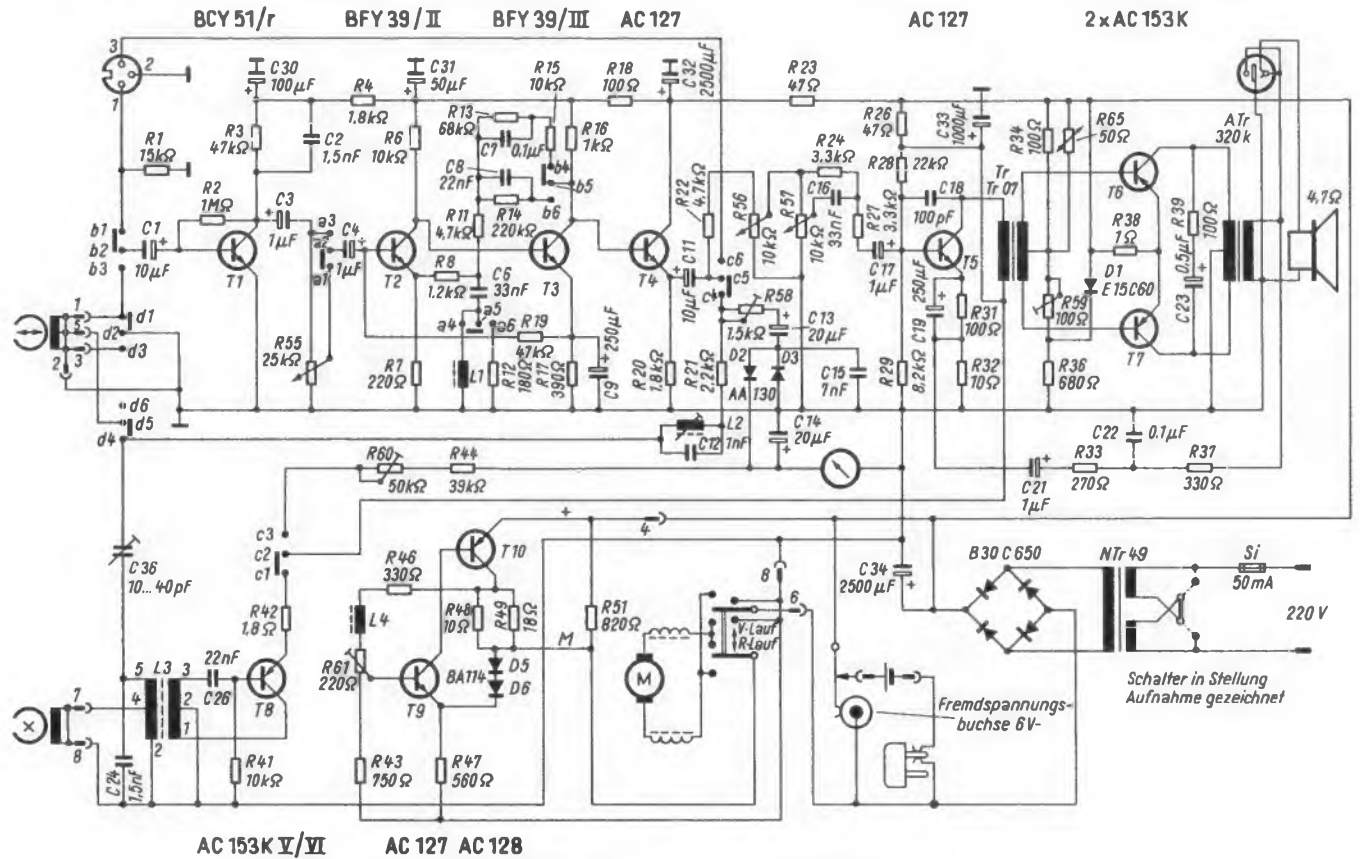
Bild 8. Gesamtschaltung des Kassetten-Tonbandgerätes Optacord 450
