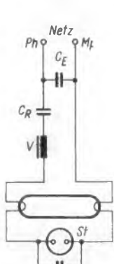
Bild 3. Entstören einer Leuchtstofflampe in kapazitiver Schaltung. Der Kompensationskondensator (hier C_R ) liegt in Reihe mit der Drossel
