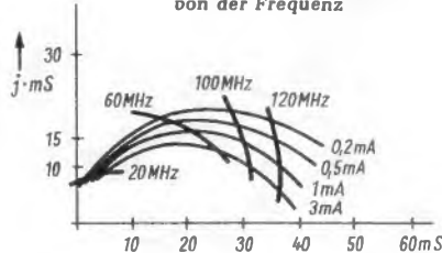
Bild 5. Ortskurvenschar für den Kurzschluß-Eingangsleitwert in Emitterschaltung für verschiedene Emitterströme
