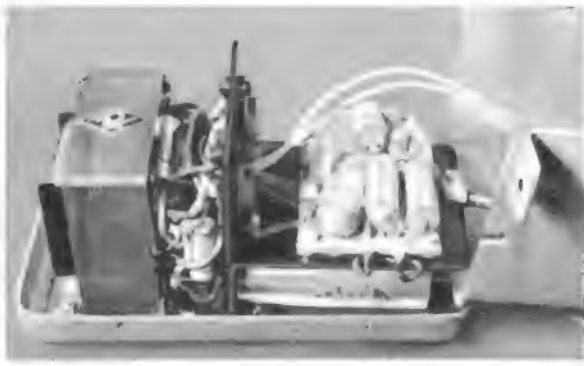
Bild 2. Ansicht der vom Verfasser gebauten Musteranlage der Thyristorzündung. Die Bauteile des Steuerteils (rechts) sind mit Kunstharz überzogen, um Störungen durch Kondenswasser zu vermeiden
