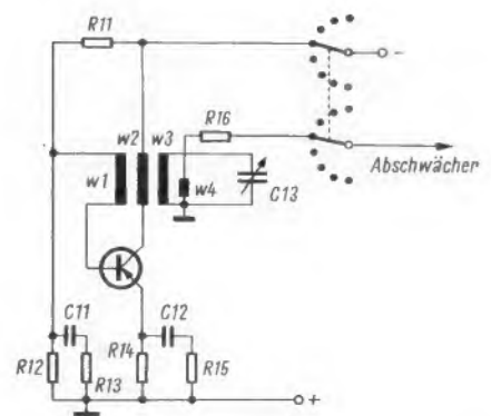
Bild 6. Schaltbild einer Oszillatorstufe als Beispiel für die Berechnung der Stabilisierungsschaltung
