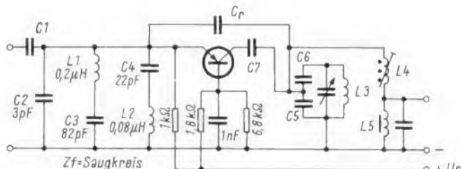
Bild 11. Prinzipschaltung einer selbstschwingenden Mischstufe
