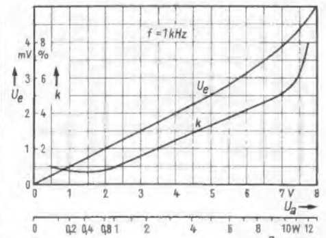
Bild 3. Empfindlichkeit und Klirrfaktor des 12-W-Verstärkers
