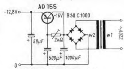
Bild 12. Netzgerät zu Bild 11
