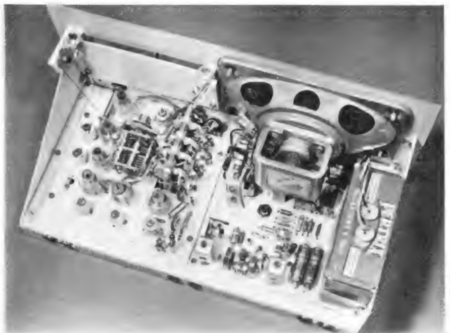
Bild 2. Chassisansicht von rückwärts
