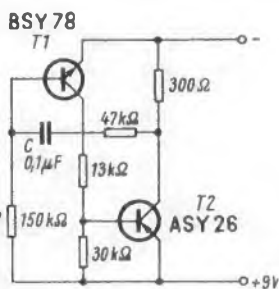
Bild 1. Impulsgenerator mit Komplementär-Transistoren; R und C sind die frequenzbestimmenden Elemente
