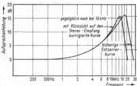
Links: Bild 3. Korrektur der Aufsprecherhöhenanhebung
