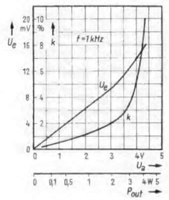
Rechts: Bild 13. Empfindlichkeit und Klirrfaktor des Gegentakt-A-Verstärkers nach Bild 11
