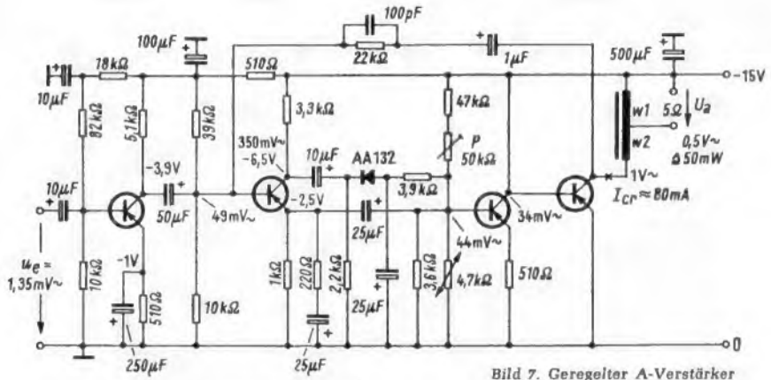
Bild 7. Geregelter A-Verstärker mit 5 W Ausgangsleistung
