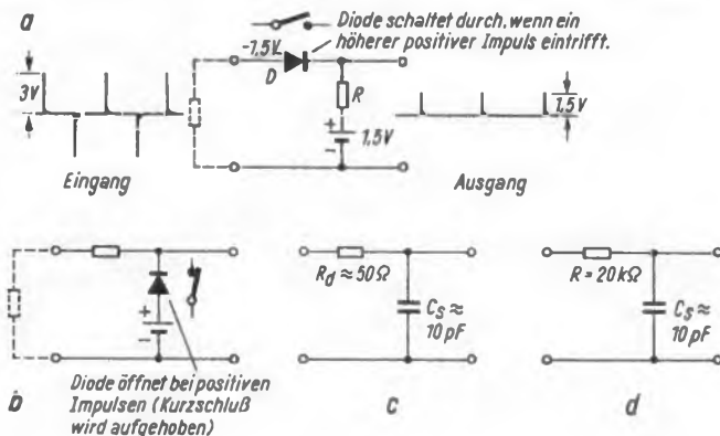
Bild 20. Diodenschalter zum Abkappen von Impulsen; a = die Diode D schaltet durch, wenn ein positiver Impuls die Vorspannung überwindet; b = der durch die Diode gebildete Kurzschluß wird durch positive Impulse aufgehoben; c = Ersatzschaltung von Bild 120a, dargestellt als Tiefpaß bei durchgeschalteter Diode; d = Ersatzschaltung für Bild 120b
