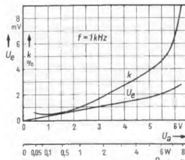
Bild 2. Empfindlichkeit und Klirrfaktor des 7-W-Verstärkers
