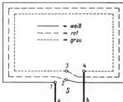
Bild 2. Vorschlag für eine Induktionsschleife aus dreifädigem Kabel
