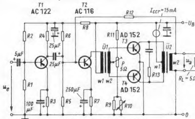
Bild 1. Gegentakt-B-Verstärker
