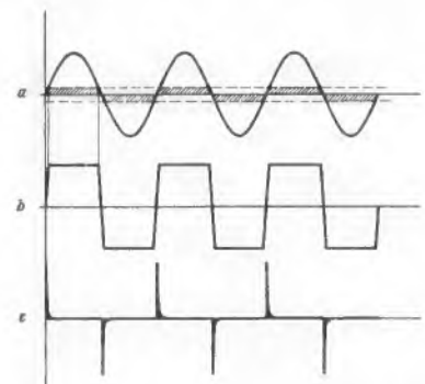
Bild 119. Bildung von Zählimpulsen aus einer Sinusschwingung. Die Sinusschwingung a wird in einer Begrenzerschaltung abgekappt. Nach dem Verstärken ergibt sich die annähernde Rechteckschwingung b. Durch Integrieren an einem CR-Glied erhält man die Nadelimpulse c. Die negativen Impulse kann man mit Hilfe einer Schaltdiode unterdrücken
