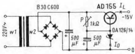
Bild 10. Stabilisiertes Netzgerät zu Bild 7
