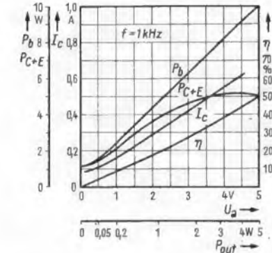
Bild 8. Verlustleistung, Kollektorstrom und Wirkungsgrad des geregelten A-Verstärkers
