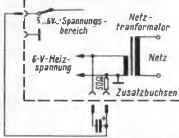
Links: Bild 1. Die Meßschaltung mit den Zusatzbuchsen für Kapazitätsmessungen
