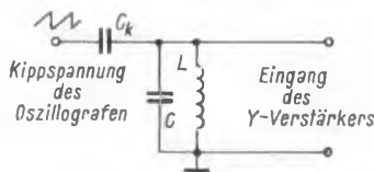
Bild 1. Einfache Oszillografen-Prüfschaltung für verdächtige Spulen
