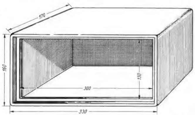
Unten rechts: Bild 6. Konstruktions-skizze für das Einschubgehäuse
