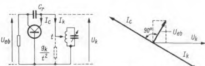
Bild 8. Oszillator mit kapazitiver Rückkopplung
