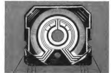
Potentiometer-Widerstandsplatte in Dünnschicht-Technik (Siemens)
