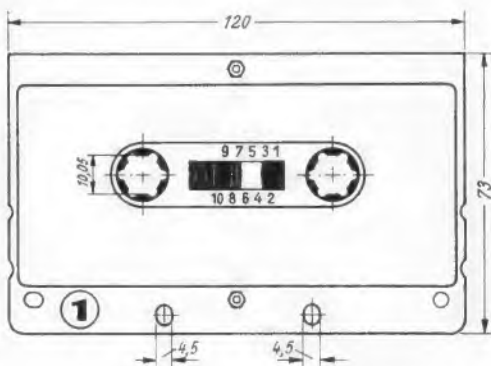
Maße der Kassette DC International
