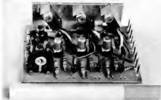
Bild 5. Der elektronische Steuerteil des Motors im Größenvergleich zu einer Zigarette
