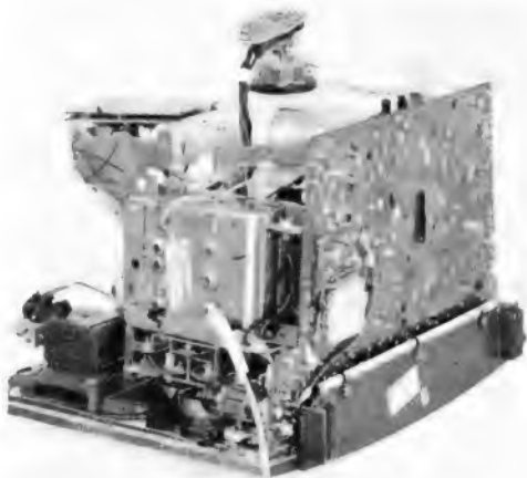
Bild 7. Blick auf das herausgenommene Chassis des Imperial-Chico. Vorn im Bild der Allbereichs-Kanalschalter T 23
