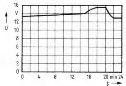
Bild 13. Letzter Teil der Ladespannungskurve der Dryfit-Batterien im Astronaut 1819 (der gesamte Ladevorgang dauert etwa zehn Stunden). Beim Abschalten fließen noch 550 mA, anschließend fließen nur noch 25 mA Nachladestrom
