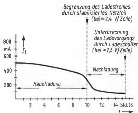
Bild 12. Ladestromkurve der Batterien im Optaport 305
