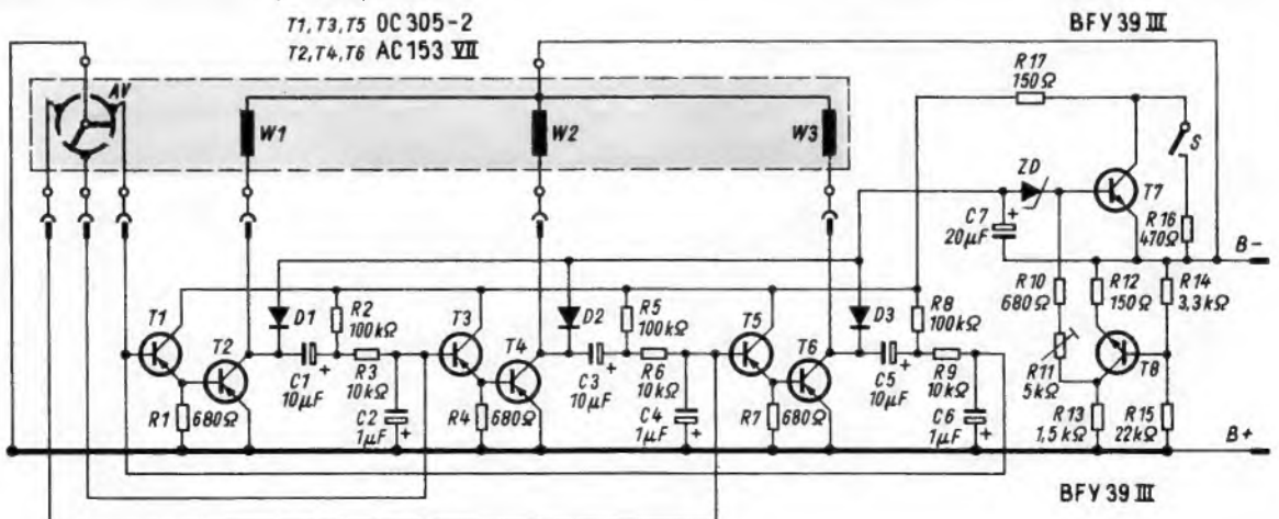
Bild 1. Schaltung des im Uher-Report-Tonbandgerät verwendeten neuen Gleichstrommotors
