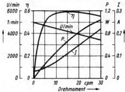
Bild 7. Leistungskurven des unregulierten Motors bei U b = 9 V; η = Wirkungsgrad, P = abgegebene Leistung, U/min = Drehgeschwindigkeit, I = aufgenommener Strom.
