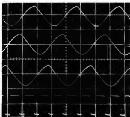
Bild 2. Verlauf der Spannungen im Leerlauf des Motors
