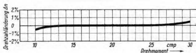
Bild 7. Drehzahländerung in Abhängigkeit vom Drehmoment bei einer Betriebsspannung von 6 V
