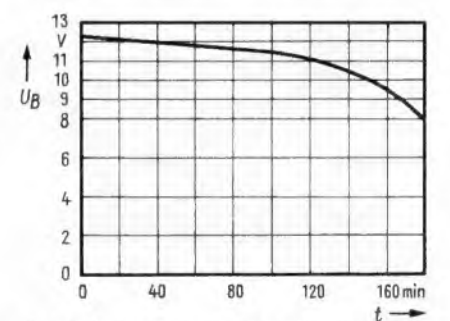
Bild 15. Entladekurve bei 2,4 A Stromentnahme
