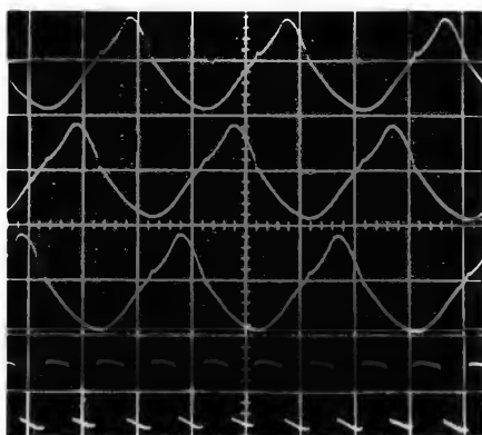
Bild 3. Spannungen bei einem Drehmoment von 25 cpm
