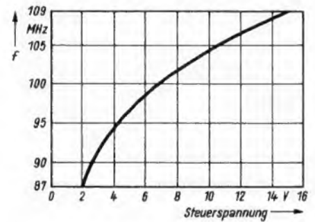
Bild 2. Frequenzvariation in Abhängigkeit von der an den Dioden anliegenden Steuerspannung
