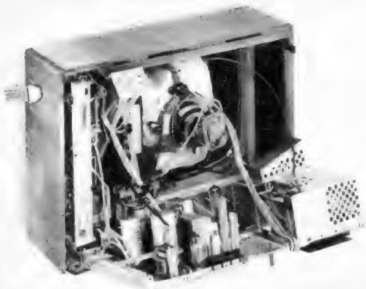
Bild 4. Klappchassis des T 105 P von Telefunken
