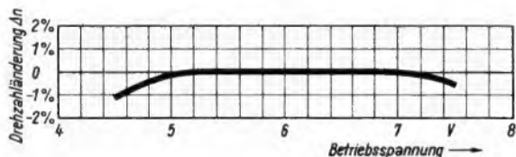
Bild 6. Drehzahländerung in Abhängigkeit von der Betriebsspannung bei einem Drehmoment von 16 cpm
