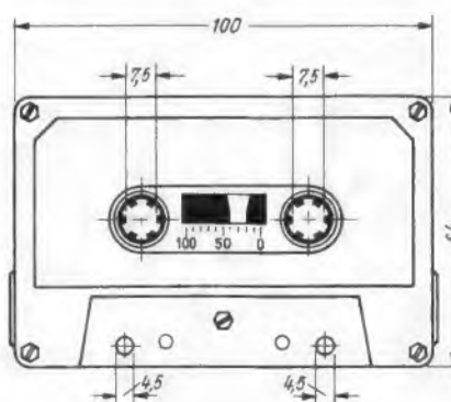
Maße der Compact-Cassette
