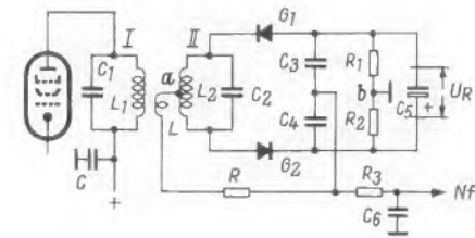
Bild 11. Gesamtschaltung des symmetrischen Ratio-Detektors
