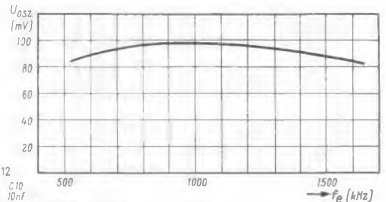
Bild 2. Verlauf der Oszillatorspannung, gemessen am Emitter, in Abhängigkeit von der Eingangs-frequenz. U_B = 2,4 V, I_C = 0,5 mA
