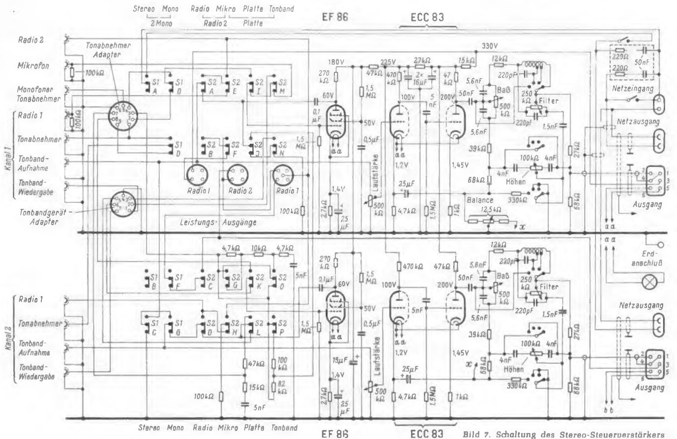
Bild 7. Schaltung des Stereo-Steuerverstärkers
