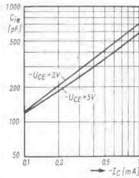
Bild 5. Eingangskapazität als Funktion des Kollektorstromes
