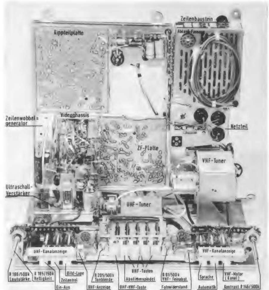
Bild 1. Chassis des Loewe-Opta-Spitzengerätes Arena 33080
