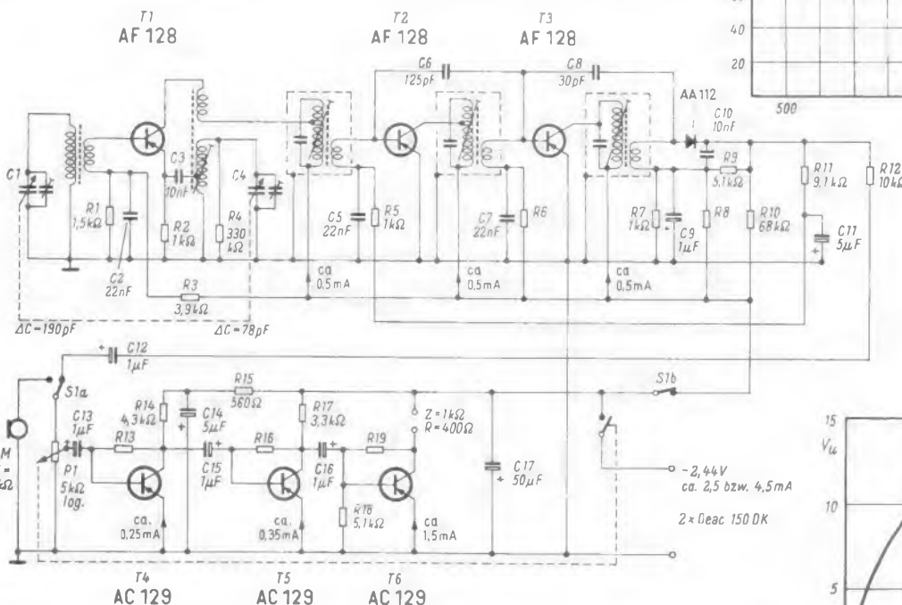
Bild 1. Schaltung des Mittelwellenempfängers mit Subminiatur-Transistoren. Folgende Widerstandswerte ändern sich entsprechend der Farbkennzeichnung der Transistoren, die deren Stromverstärkungsfaktor angibt: rote Farbgruppe: R 13 = 91 k \Omega , R 16 = 91 k \Omega , R 19 = 13 k \Omega ; gelbe Farbgruppe: R 6 = 240 k \Omega , R 8 = 10 k \Omega , R 13 = 150 k \Omega , R 16 = 150 k \Omega , R 18 = 18 k \Omega , R 19 = 18 k \Omega ; blaue Farbgruppe: R 6 = 470 k \Omega , R 8 = 15 k \Omega , R 13 = 330 k \Omega , R 16 = 330 k \Omega , R 19 = 24 k \Omega
