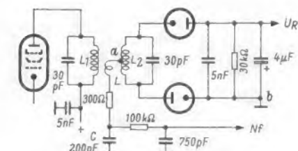
Bild 18. Unsymmetrische Schaltung des Ratio-Detektors
