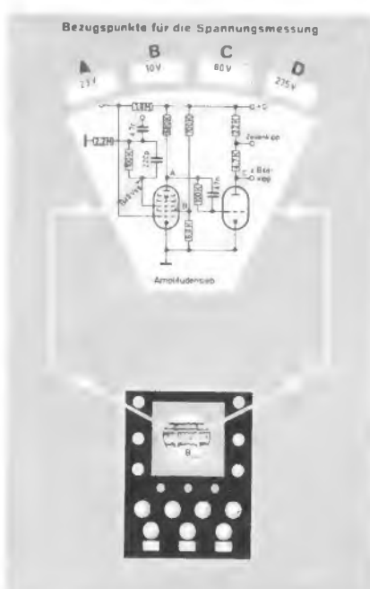
Bild 2. Die Rückseite der gleichen Einstellung. Oben die Teilschaltung der Stufe mit Spannungsangaben, unten ein typisches Oszillogramm
