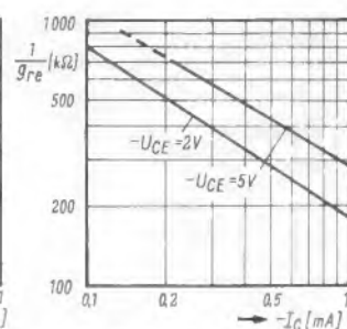
Bild 8. Rückwirkungswiderstand als Funktion des Kollektorstromes
