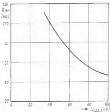
Bild 3b. Mischer-Innenwiderstand für die Zwischenfrequenz als Funktion der Oszillatorspannung. Daten wie in Bild 3a
