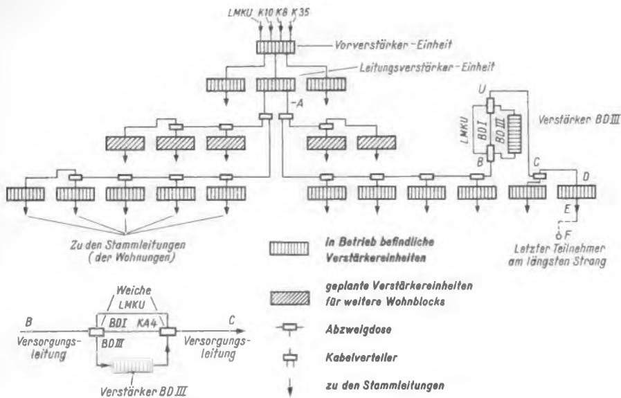
Bild 3. Schaltschema der Gemeinschaftsantennen-Anlage
