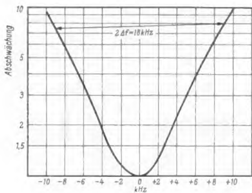
Links: Bild 11. Zf-Selektionskurve, gemessen ab Basis der Mischstufe, f_z = 455 \text{ kHz}
