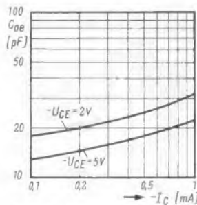
Bild 7. Ausgangskapazität als Funktion des Kollektorstromes
