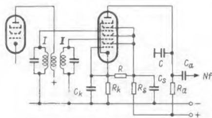
Bild 21. Schaltung des Phasenwinkeldetektors mit der Röhre EQ 80
