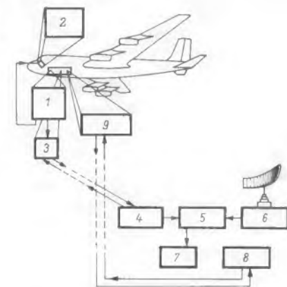
Bild 2. Schema der HARCO-Anlage; 1 = Bord-navigationsanlage mit digitalem Ausgang, 2 = bildliche Darstellung für den Piloten, 3 = Bord-Datenübertragungsanlage, 4 = Boden-Datenüber-tragungsanlage, 5 = Rechnergerät, 6 = Radar, 7 = Verkehrslage-Darstellung, 8 = Sprechfunk-oberbindung vom Boden, 9 = Sprechfunkverbin-dung von Bord
