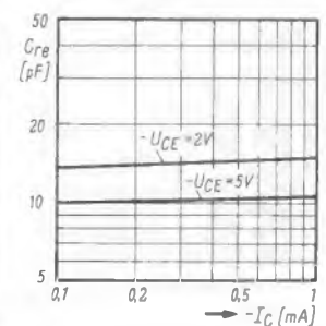
Bild 9. Rückwirkungskapazität als Funktion des Kollektorstromes
