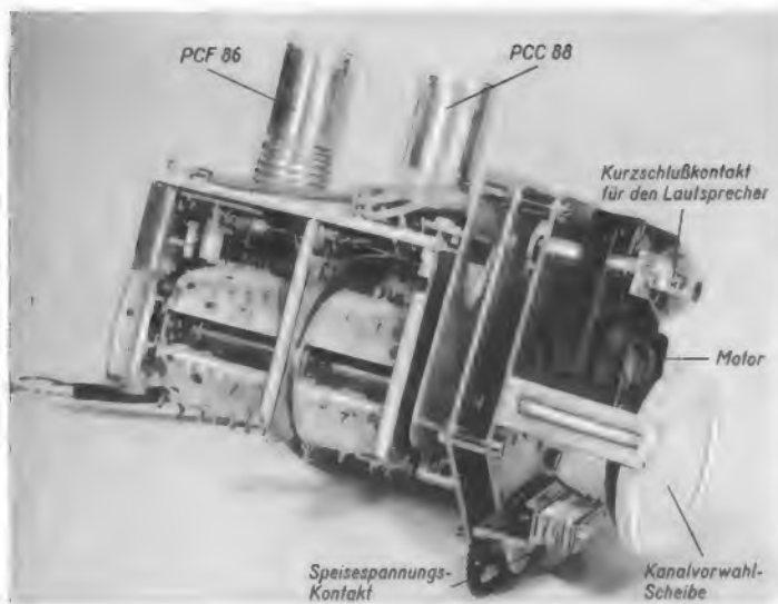
Bild 2. VHF-Kanalschalter mit Motorantrieb
