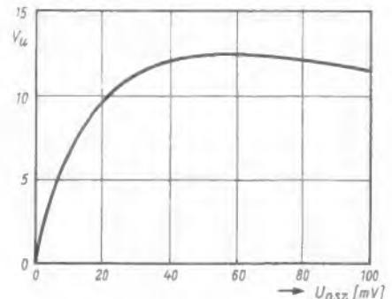
Unten: Bild 3a. Mischverstärkung als Funktion der Oszillatorspannung, gemessen bei U_B = 2,4 V, -I_C = 0,5 mA, f_e = 1 MHz, f_z = 455 kHz, Zf-Last = 1 k \Omega
