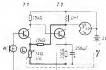
Bild 3. Die Schaltung des eingebauten Vorverstärkers; T1 = T2 = OC 305/1
