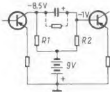
Bild 1. Wirkung des Isolationswiderstandes von Koppelkondensatoren zwischen zwei Transistoren
