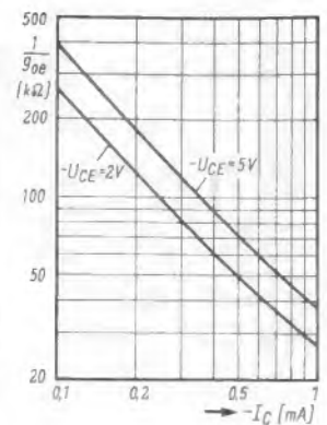
Bild 6. Ausgangswiderstand als Funktion des Kollektorstromes
