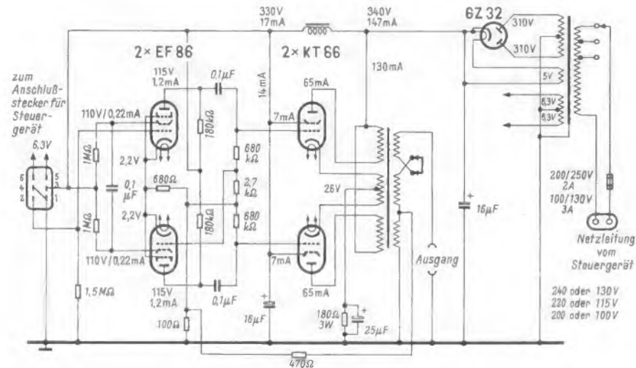
Bild 4. Schaltung des Endverstärkers
