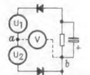
Bild 19. Das Brückenprinzip beim unsymmetrischen Ratio-Detektor
