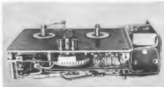
Unten: Bild 33. Das fertige Gerät von der Seite gesehen Rechts: Bild 34. Frontplatte mit Bedienungssteil vor dem Einbau in das Gehäuse
