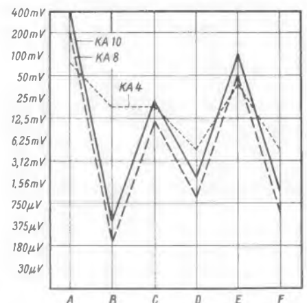
Bild 4. Spannungsverlauf der Kanäle 10, 8 und 4 nach Inbetriebnahme der Anlage. Die Tabelle nennt die Hochfrequenzspannungen in mV, gemessen an den Punkten A bis F in Bild 3
