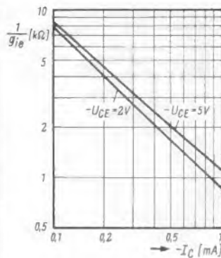
Bild 4. Eingangswiderstand als Funktion des Kollektorstromes
