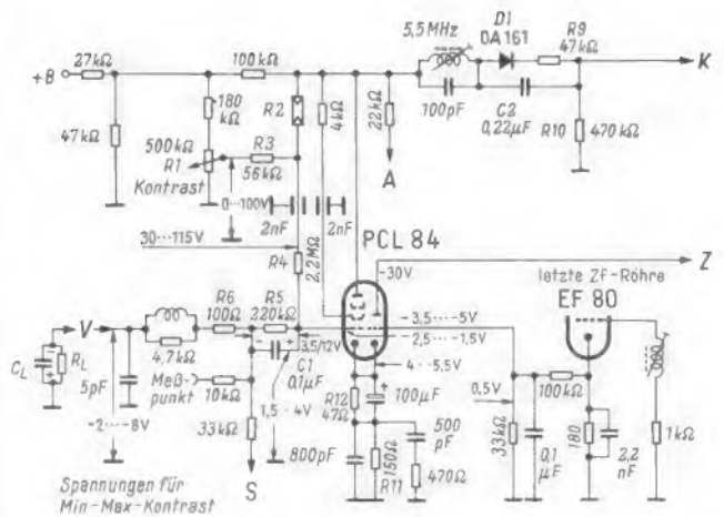
Bild 4. Schaltung der Video-Endstufe. A = Amplitudensieb, K = Katode der Bildröhre, S = Störaustattung, V = Videodiode, Z = Zeilenrücklaufimpuls und Regelspannung
