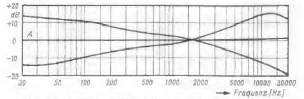
Bild 8. Frequenzgang des Baß- und des Höheneinstellers; A = Mittelstellung (linear)
