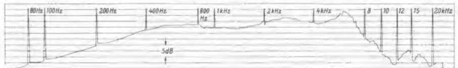
Bild 2. Frequenzkurve des Babysitter-Mikrofons; maßstäblich abgezeichnete Registrierstreifen eines Tonfrequenz-Pegelschreibers. Die hohen Zacken sind keine Resonanzstellen im Mikrofon, sondern automatisch eingblendete Frequenzmarken (nach einer Messung von Sennheiser electronic)
