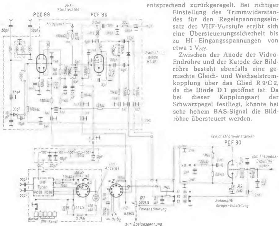
Bild 3. Schaltung des VHF-Kanalschalters mit automatischer Scharfjustierung
