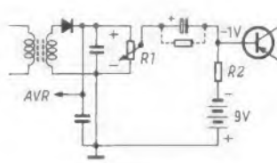
Bild 2. Prinzipschaltung der Kopplung zwischen Demodulator- und erster NF-Stufe
