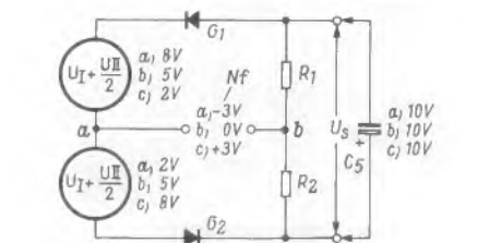
Bild 16. Anwendung des Brückenprinzips auf den Ratio-Detektor. Der Kondensator C 5 hat keinen Einfluß auf die Niederfrequenz (Ersatzschaltung des Ratio-Detektors)
