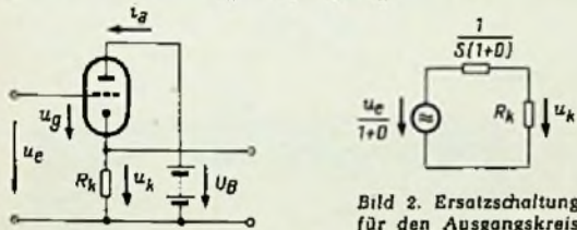
Bild 1. Grundschaltung des Katodenverstärkers: i_a = Anodenwechselstrom, u_a = Anodenwechselspannung, u_k = Katodenwechselspannung (Ausgangswechselspannung), u_e = Eingangswchselspannung, u_g = Gitterwechselspannung
