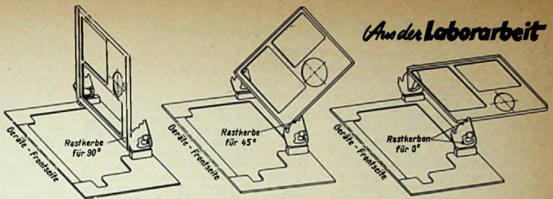
Bild 3. Klapp-Chassis der Loewe-Opta-Geräte in Gebrauchs-Stellung
