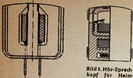
Bild 4. Schnitt durch einen Doppelspur-Ferrit-Löschkopf
