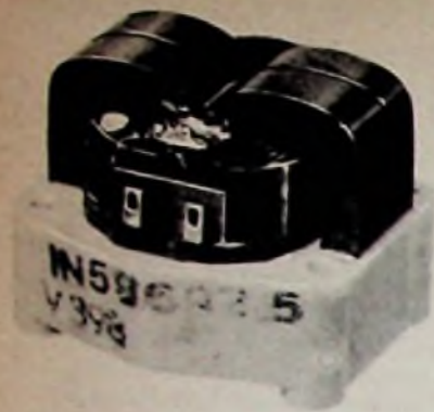
Bild 3. Valvo-Ausgangstransformator für Vertikal-Ablenkung Typ AT 3506
