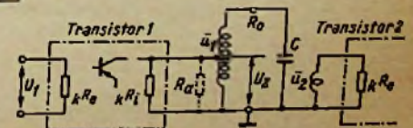
Bild 2. Zur optimalen Anpassung kR_i an kR_e über die zugeordneten Übersetzungsverhältnisse \bar{u}_1 und \bar{u}_2
