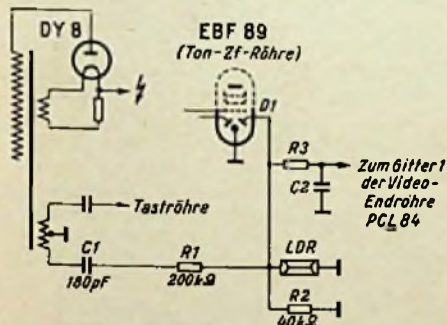
Bild 1. Schaltung der Raumlicht-Automatik mit LDR-Widerstand
