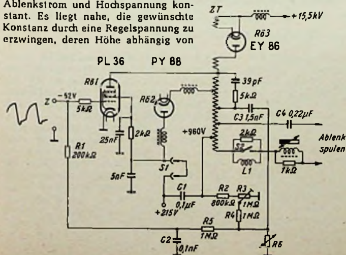
Bild 1. Zeilenkipp-Endstufe mit Bildbreitenstabilisierung
