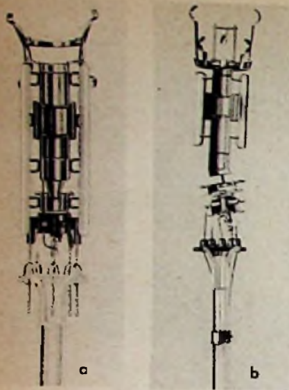
Bild 4. Schnittbilder von Bildröhrensystemen; a = Tetrodensystem der 110°-Röhren, b = Pentodensystem der 90°-Röhren
