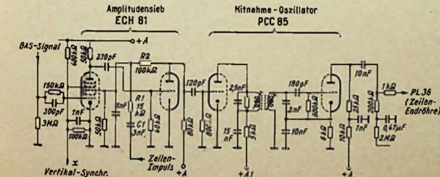
Bild 3. Zeilenablenkschaltung (ohne Endstufe); als Mitnahmeoszillator dient die Röhre PCC 85 mit vorgegeschaltetem getastetem Amplitudensieb mit der Röhre ECH 81
