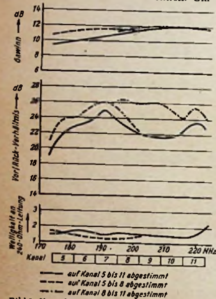
Bild 3. Kenndaten der Hochleistungs-Breitband-Antenne Fesa 14 F
