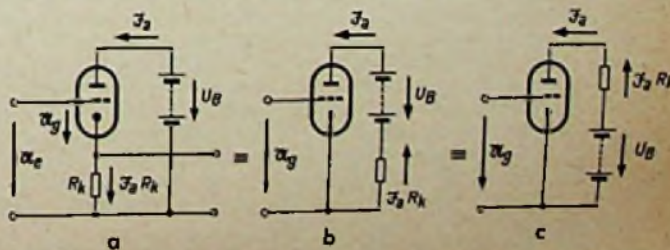
Bild 4. Verlegung des Arbeitswiderstandes auf die Anodenseite
