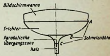
Bild 2. Seitenansicht des Kolbens
