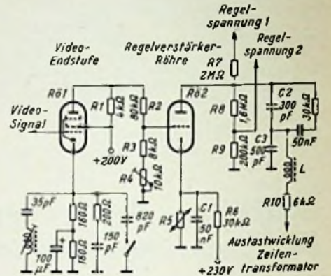
Bild 7. Schaltung zur Schwarzpegelhaltung
