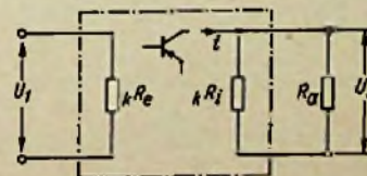
Bild 1. Zur optimalen Anpassung wird kR_i = R_a gemacht
