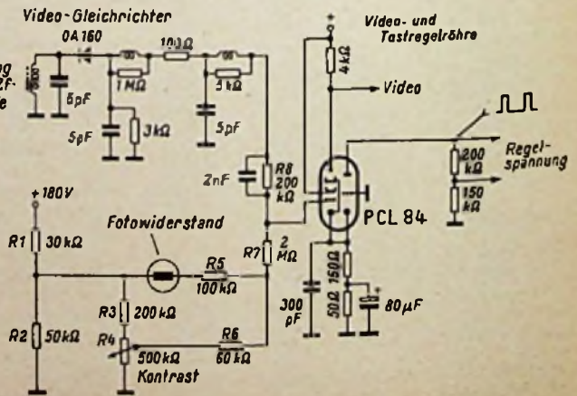
Bild 2. Automatische Kontrastregelung
