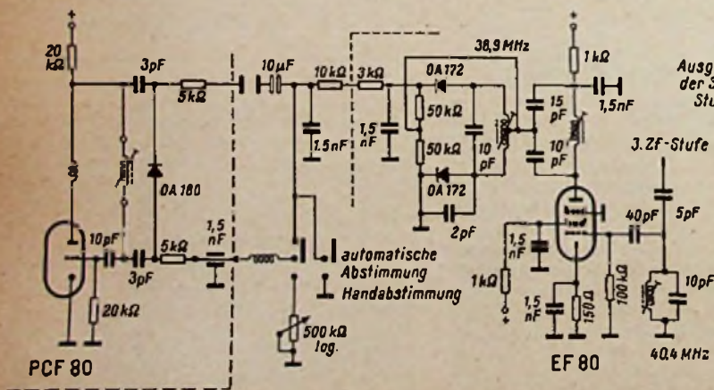
Bild 1. Schaltung der automatischen Feinabstimmung bei den Loewe-Opta-Geräten
