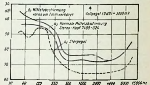
Bild 9. Übersprechdämpfung des Stereo-Kopfes bei V = 19,05 cm/sec
