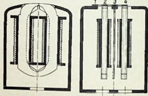
Bild 7. Viertelspur-Stereokopf
