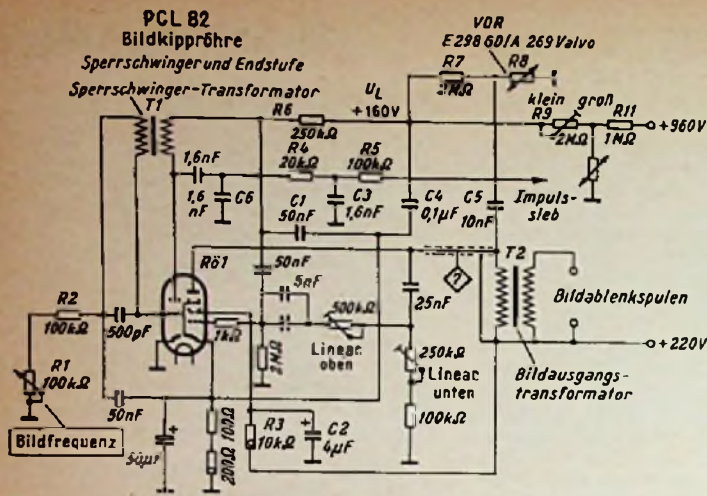
Bild 5. Bildkipp-Endstufe mit Bildhöhenstabilisierung
