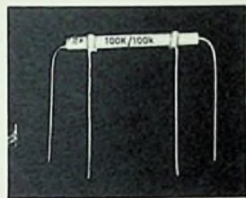
Bild 2. Praktische Ausführung einer RC-Kombination
