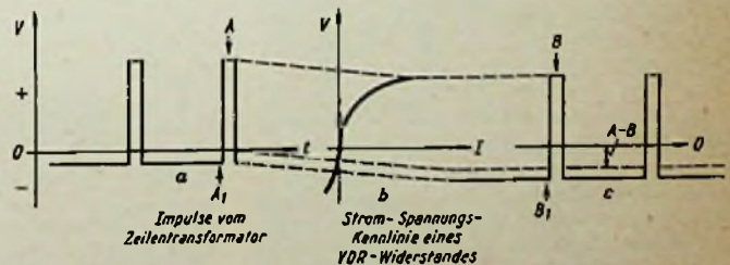
Bild 3. Rücklauf-Impulse am Zeilentransformator
