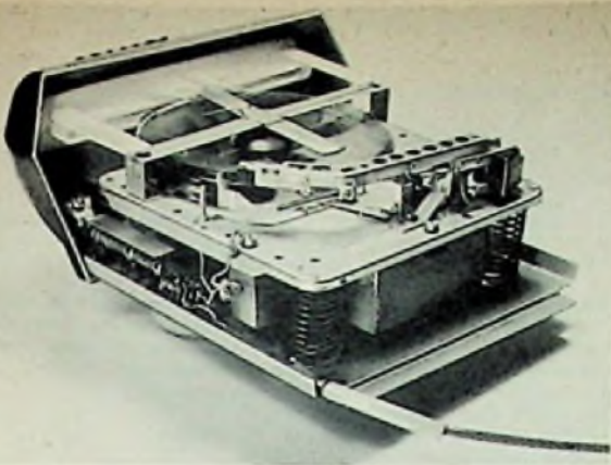
Bild 1. Chassis des Auto-Mignon von Philips. Man erkennt unter der Grundplatte zwei der insgesamt drei Druckfedern
