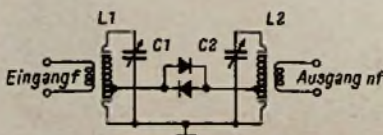
Bild 2. Frequenzverdreifachung durch Verzerrung der Kurven
