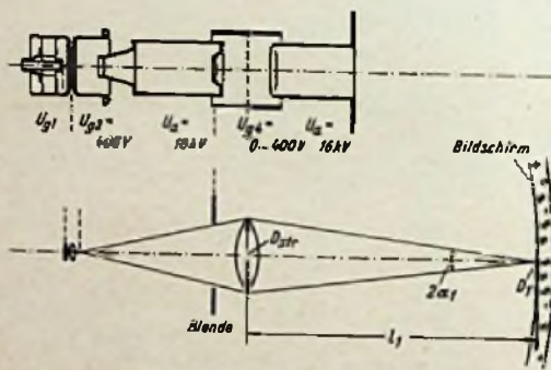
Bild 5. Schnittmodell und Strahlverlauf des 110°-Systems
