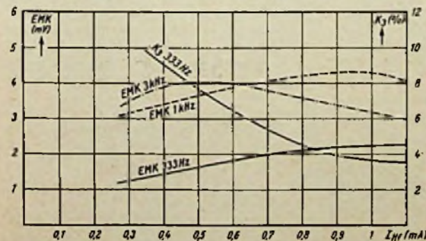
Bild 4. Halbspur-Stereokopf; Differentialkurven für DIN-BB-Leerteil, V = 9,5 \text{ cm/sec} , I_{HH} = 0,08 \text{ mA} = \text{const} , f_{HH} = 45 \text{ kHz}
