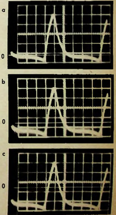
Bild 4. Die Abhängigkeit der Öffnungszeit des Amplitudensiebs Bild 3 von der Nullpunktage; a = unvollständig integrierter Tastimpuls bei großer Öffnungszeit, b = mittlere Öffnungszeit, c = kleine Öffnungszeit
