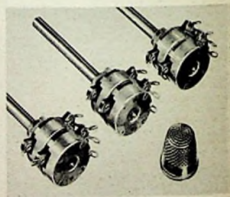
Bild 13. Valvo-Kleinpentiometer für Stereo-Verstärker
