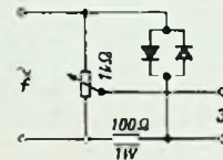
Bild 3. Erzeugung von Oberschwingungen durch Gleichrichtung beider Halbwellen
