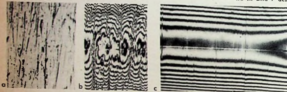
Bild 8. Aufnahmen der Lauflinien von Tonköpfen; a = normale Mikroskop-Aufnahme nach dem Vorschleiff; b = gleiches Bearbeitungsstadium wie a, aufgenommen mit dem Interferenz-Mikroskop; c = Interferenz-Aufnahme nach der End-Bearbeitung, der Tonspalt ist als horizontale Mittellinie zu erkennen, rechts am Rand eine restliche Bearbeitungsspur von 0,2 \mu Breite
