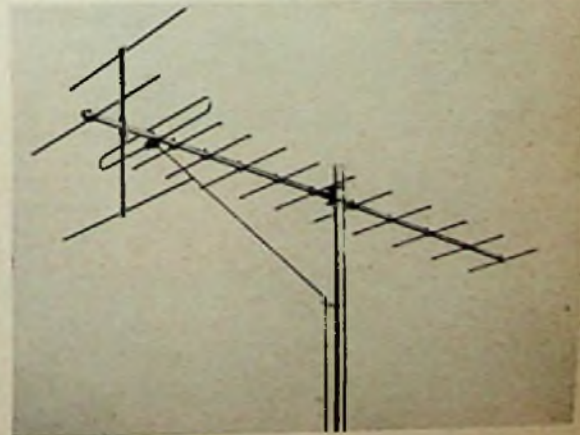
Bild 2. Hochleistungs-Breitband-Antenne Fesa 14 F. Sie ist durch Biegeenden auf das gesamte Fernsehband III oder auf die untere oder die obere Bandhälfte abstimbar
