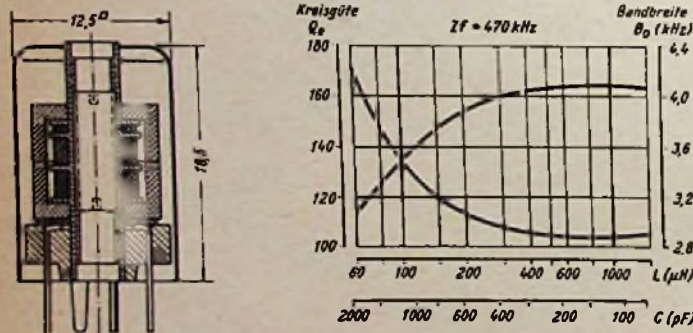
Bild 4. Kreisgüte Q_0 (rechts ansteigend), Bandbreite B_0 (rechts abfallend) in Abhängigkeit von der Induktivität L und der Kapazität C für den Zf-Kreis D 31 A. Zf = 470 \text{ kHz}
