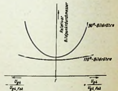
Bild 6. Relativer Bildpunktdurchmesser in Abhängigkeit von der Linsenspannung U_{g4}/U_{g4, fok} . Darin ist U_{g4, fok} = Fokussierspannung
