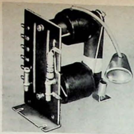
Bild 4. Valvo-Ausgangstransformator für Horizontal-Ablenkung Typ AT 2016/20
