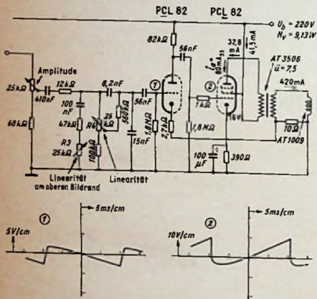
Bild 6 eine Schaltung mit Strom-Gegenkopplung. In Bild 3 ist ein Vertikal-Transformator in Bandwickeltechnik aus Textur-Eisen wie der gegeben. Er ist kleiner und leichter als bisher übliche Transformatoren dieser Art.
