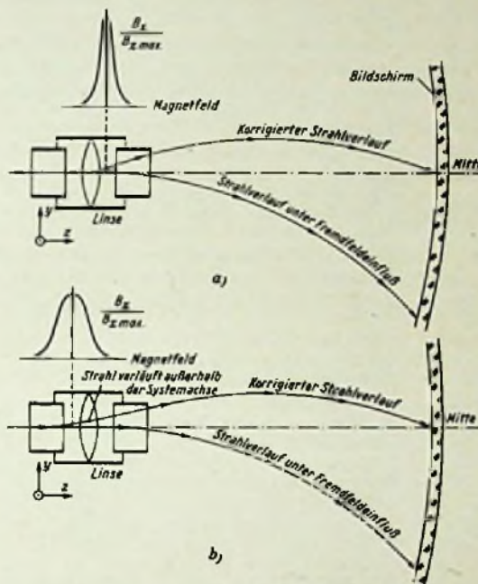
Bild 8. Korrektur des vorabgelenkten Elektronenstrahls durch den Zentriermagneten; a = Richtige Lage des Zentriermagneten, b = Falsche Lage und falsche Feldform des Zentriermagneten (schematische Darstellung)
