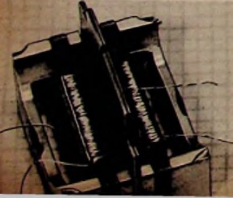
Bild 8. Viertelspur-Stereokopf; Kernpakete mit Wicklung im Halterahmen mit Zwischenabschirmung
