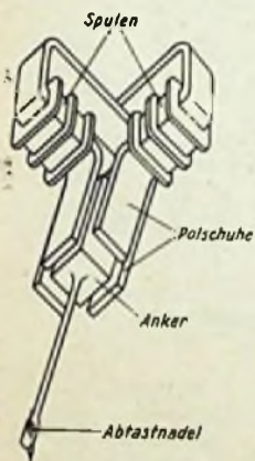
Bild 1. Schematischer Aufbau des Stereo-Tonabtasters STS 300
