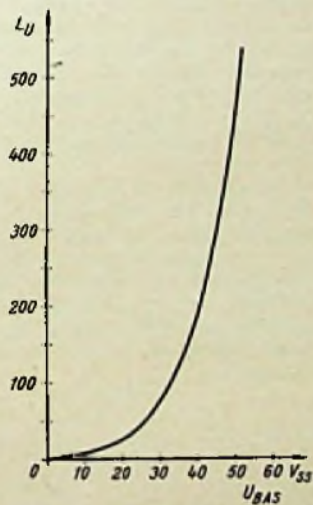
Bild 2. Ansteigen der Videospannung an der Bildröhrenkathode in Abhängigkeit von der Leuchtdichte des Umfeldes ( L_U ) des Bildschirms
