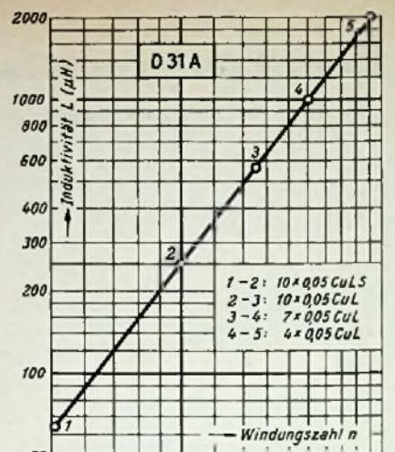
Bild 5. Die Wickelkurve für D 31 A
