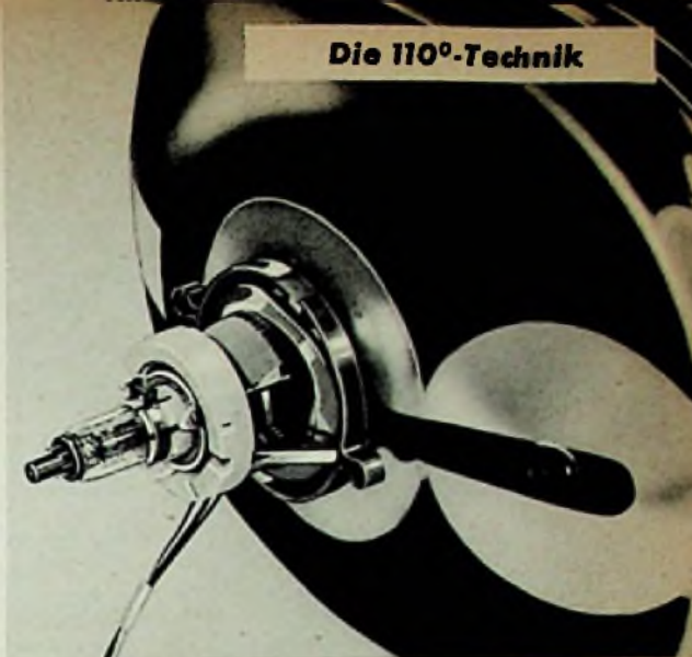
Eine 110°-Bildröhre mit aufgesetzter Ablenkeinheit Typ KE 59 (Telefunken)
