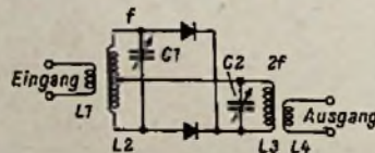
Bild 1. Frequenzverdopplung durch Zweiweggleichrichtung
