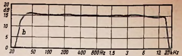
Bild 5. Ober-Aller-Frequenzgänge des Magnetophons 85; a = v = 19 cm/sec, b = v = 9,5 cm/sec
