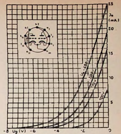
J_a = f(U_g) U_a = \text{Parameter}
