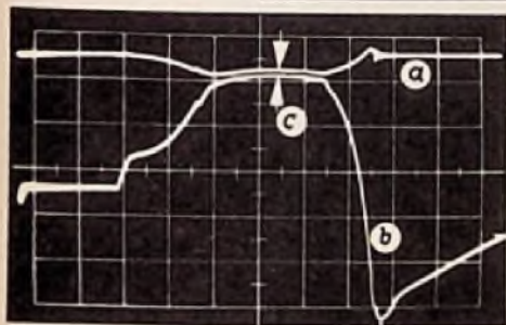
Bild 3. Doppelstrahl-Oszillogramm einer Transistor-Messung. Meßobjekt ist ein Schalt-Transistor in einer Sperrschwingler-Schaltung. a = Emittor-Spannung, b = Kollektor-Spannung.
