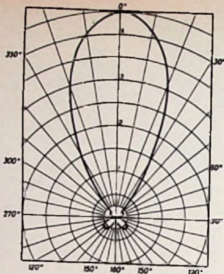
Bild 6. Horizontalcharakteristik der Feso 22 0 bei 495 MHz - Kanal 15
