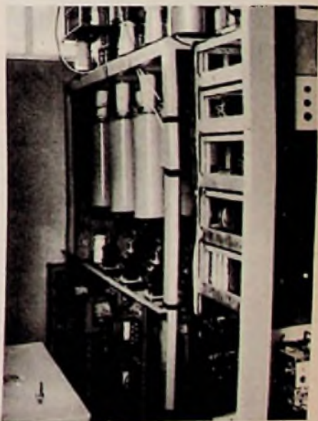
Bild 3. In den senkrechten Zylindern befinden sich die zum ersten Male benutzten Silizium-Hochspannungsgleichrichter
