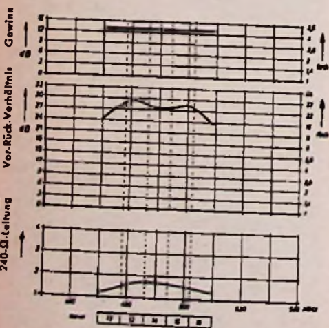
Bild 7. Gewinn, V/R-Verhältnis und Welligkeit in den Kanälen 12 bis 16 für die 22-Elementantenne nach Bild 5
