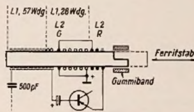
Bild 5. Anordnung der Spulennicklungen
