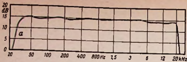
Bild 5. Ober-Aller-Frequenzgänge des Magnetophons 85; a = v = 19 cm/sec, b = v = 9,5 cm/sec
