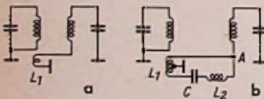
Bild 1. Schaltung des Zf-Verstärkers, Videogleichrichters und Videoverstärkers bei den Graetz-Empfängern Fährnich, Markgraf und Mandarin
