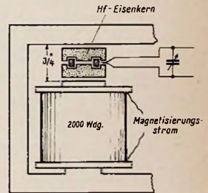
Bild 3. Mechanische Anordnung der Prinzipschialtung Bild 1. Im erweiterten Luftspalt eines Transformator-kernes aus M-Bleichen liegt der Hf-Eisenkern
