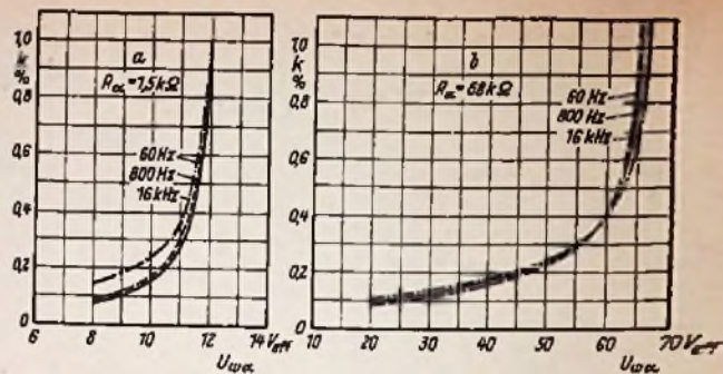
Bild 12. Klirrfaktor als Funktion der Ausgangsspannung in Schalterstellung 20 Hz...100 kHz. a für R_a = 1,5 \text{ k}\Omega , b für R_a = 68 \text{ k}\Omega
