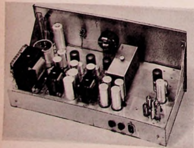
Bild 15. Chassis-Unterseite des Meßverstärkers (Bodenplatte entfernt)
