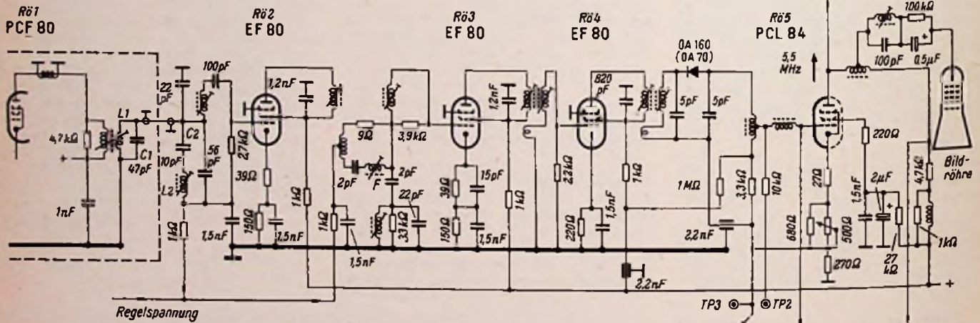
Bild 1. Schaltung des Zf-Verstärkers, Videogleichrichters und Videoverstärkers bei den Graetz-Empfängern Fährnich, Markgraf und Mandarin
