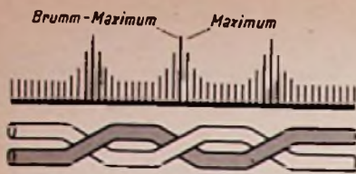
Bild 5. Vorlauf der induzierten Spannung bei einer oerdrillten Leitung
