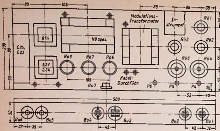
Bild 19. Modulator-Chassis
