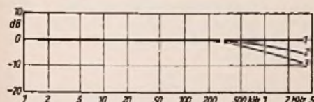
Bild 6. Frequenzgang des Ausgangsspannungsmessers bei hohen Frequenzen. Kurve 1 = endgültige Bemessung im 12- und 60-V-Bereich; Kurve 2 = C 62 weggelassen; Kurve 3 = C 61 und C 62 weggelassen
