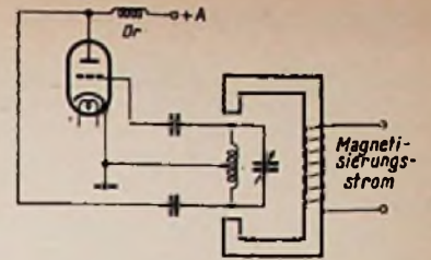
Bild 1. Prinzipschialtung eines Magnet-Variometers aus dem Jahre 1938
