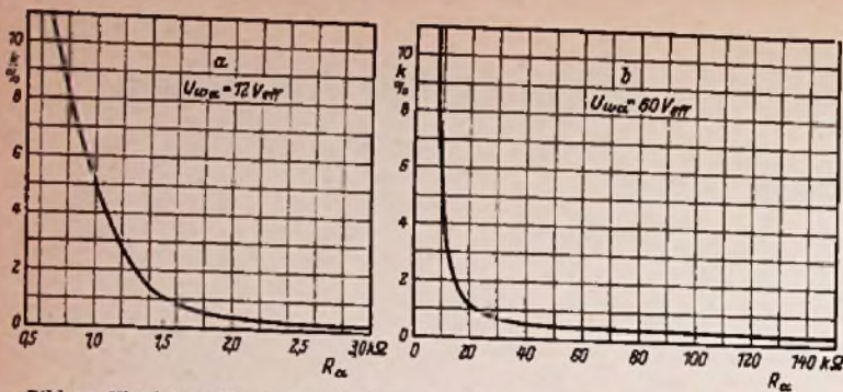
Bild 11. Klirrfaktor für 800 Hz als Funktion des Ausgangsbelastungswiderstandes in Schalterstellung 20 Hz...100 kHz; a = bei U_{\text{eff}} = 12 \text{ V} , b bei U_{\text{eff}} = 60 \text{ V}
