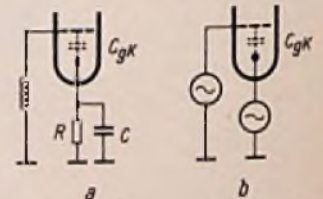
Bild 3. Schaltung zur Vermeidung von Dämpfungsänderungen im Zf-Verstärker durch den Regelvorgang. a = Schaltung, b = Prinzip
