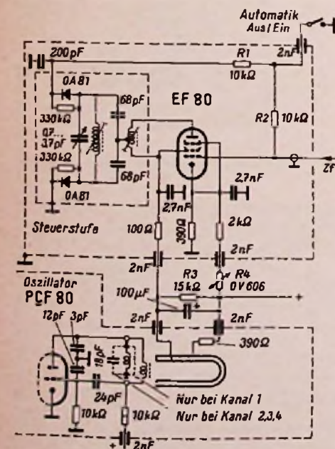
Bild 8. Nachstimmstüverschaltung von Grundig mit Magnetvariometer
