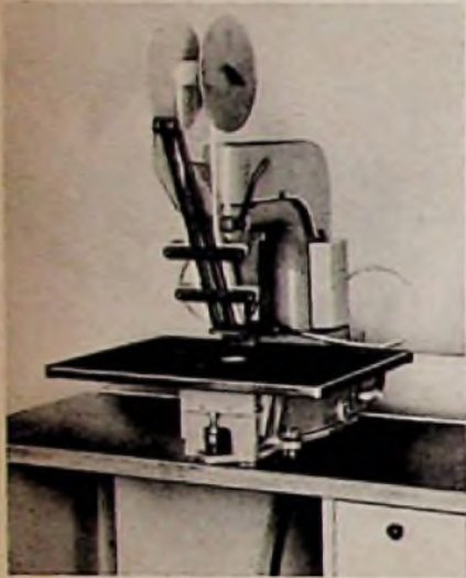
Bild 1. Dynosert-Halbautomat
