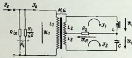
Bild 8. Stereodyn-Schaltung. Strom- und Spannungsverhältnisse, sowie Lage der Belastungswiderstände. Der Lautsprecher R_1 wurde auf die Primärseite übersetzt, um die Rechnung zu vereinfachen
