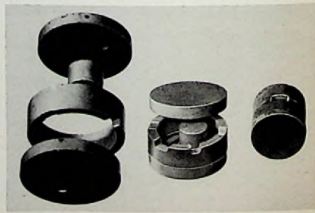
Bild 5. Topfkerne mit zwei Ringen (ganz rechts) und einem Ring (links und Mitte)
