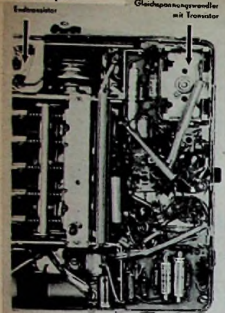
Bild 2. Teilansicht des Chassis von unten
