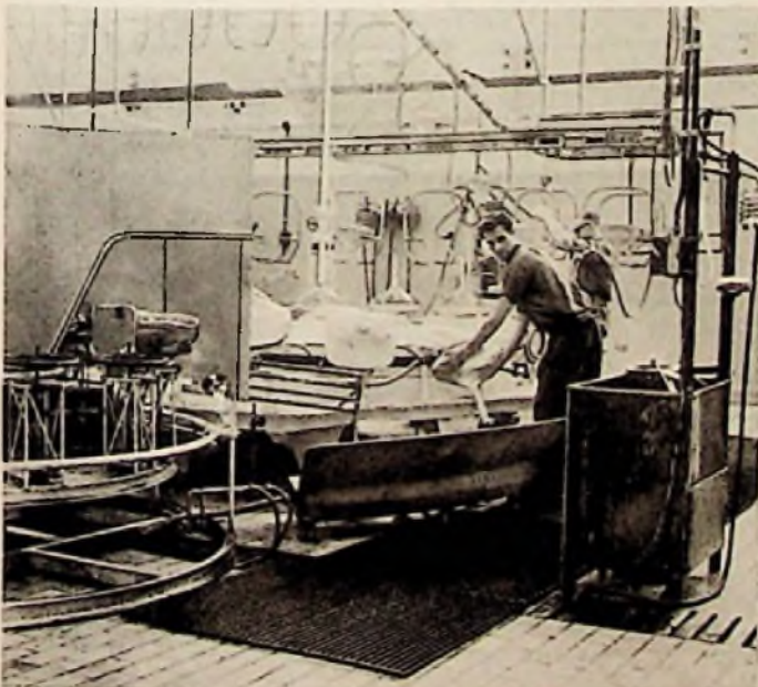
Rechts im Bild Aufbringen des Leuchtstoffes auf den Bildschirm mit einer mössorigen Suspension; links ist ein Karussell sichtbar, auf dem der Leuchtstoff ausgetrocknet wird
