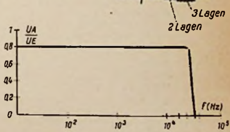
Bild 5. Frequenzgang des Tiefpaßfilters
