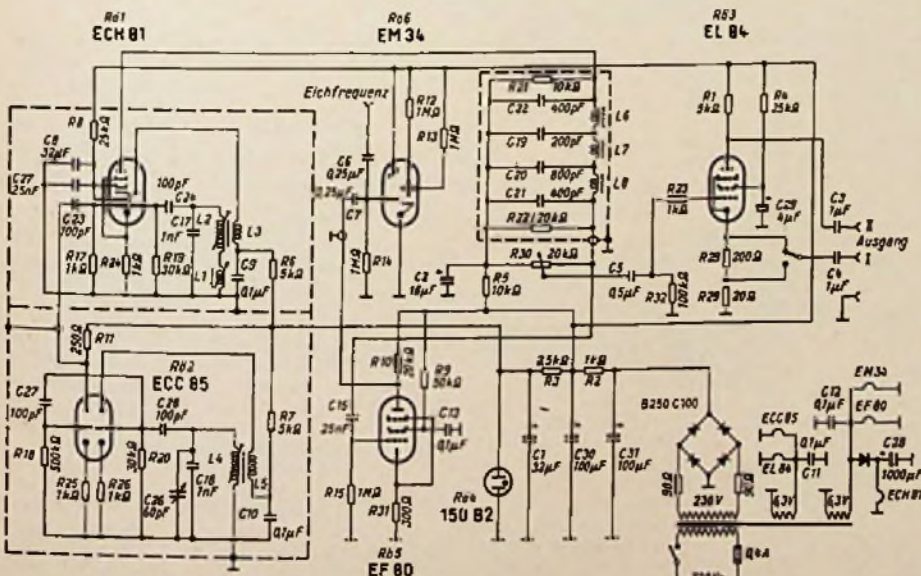
Bild 2. Schaltbild
