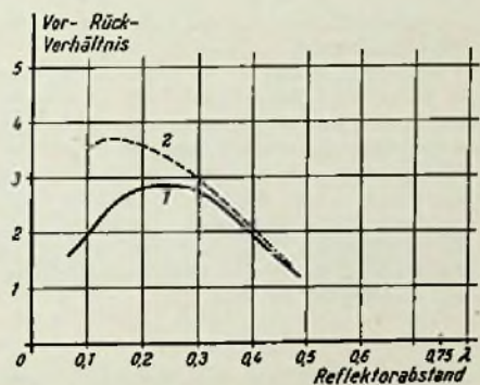
Bild 1. Die Abhängigkeit des Spannungsgewinns und des Vor-/Rückverhältnisses vom Reflektorabstand einer Fernsehantenne. Die ausgezogenen Linien 1 entsprechen dem höchsten Spannungsgewinn, die gestrichelten Linien 2 dem höchsten Vor-/Rückverhältnis
