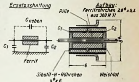
Bild 3. Praktische Ausführungsform eines Durchführungselementes; links daneben nochmals die Ersatzschaltung mit den gleichen Bezeichnungen
