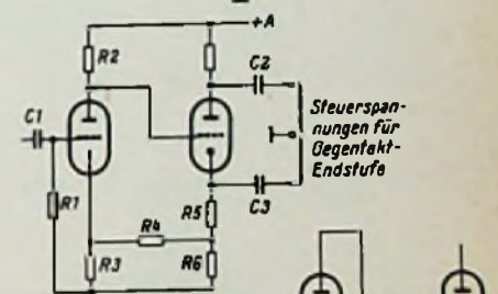
Bild 1. Rückkopplung von Katode zu Katode eines Nf-Verstärkers
