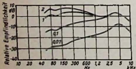
Bild 2. Änderung der Frequenzkennlinie unter dem Einfluß verschiedener Werte des Widerstandes R 1 (0,01 - 0,1 - 1 - 2 M \Omega )
