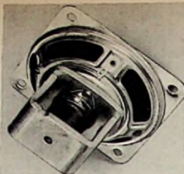
Bild 4. Lautsprecherchassis Type 49 242 42 von Valvo mit 140 \Omega Schwingungspulenimpedanz für Transistorverstärker
