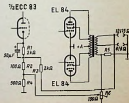
Bild 8. Kombinierte Rück- und Gegenkopplung vom Ausgang auf die Spannungsverstärkerstufe
