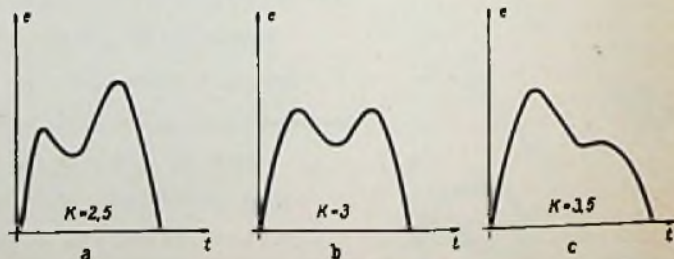
Bild 7. Verlauf der Regelpulsspannung für verschiedenes Verhältnis K der Zeilenrücklauf Frequenz zur Abstimmfrequenz der Hochspannungswicklung
