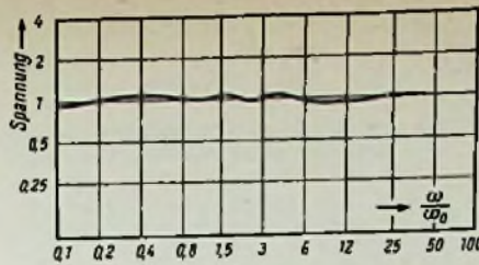
Bild 9. Verlauf der Spannung (Betrag) am Lautsprecher R_2 (Bild 8) bei Stereo-Betrieb in Abhängigkeit von der Frequenz, nach Gleichung (8) errechnete Werte. Normierte Darstellung. U_{R_2} ist der Spannungsbetrag, welcher bei Normalbetrieb an R_2 liegt. \omega_0 ist die Übergangsfrequenz der Stereodyn-Schaltung; sie beträgt im praktischen Fall z. B. 2\pi \cdot 460 Hz
