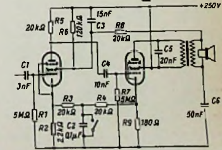
Bild 3. Frequenzabhängige Rückkopplung von Katode zu Katode
