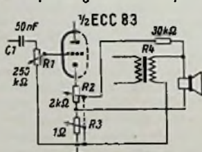
Bild 10. Gekoppelte Einstellung von Rück- und Gegenkopplung vom Ausgang auf die Katode der Spannungsverstärkerstufe
