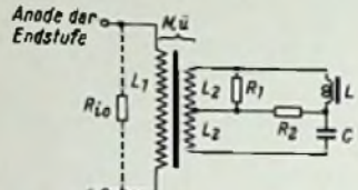
Bild 7. Stereodyn-Schaltung, Stereo-Betrieb herausgezeichnet
