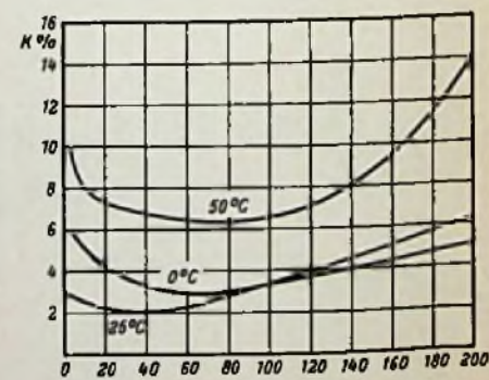
Bild 5. Zusammenhang zwischen Klirrfaktor, Ausgangsleistung und Umgebungstemperatur (10, + 25, + 50° C)
