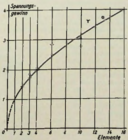
o Einkanalantennen Band III + Breitbandantennen Band III und Einkanalantennen Band I gamma Yagi mit höchstem Gewinn nach Fishenden
