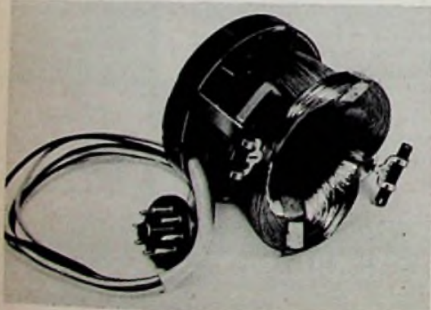
Bild 2. Die Ablenkspule
