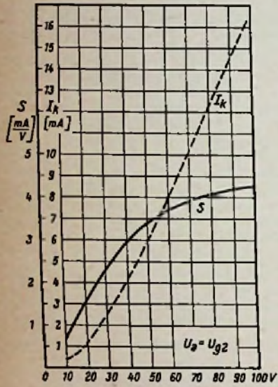
Bild 3. Steilheit S und Katodenstrom I_k in Abhängigkeit von Anoden- u. Schirmgitterspannung, gemessen an einem Exemplar der EF 83
