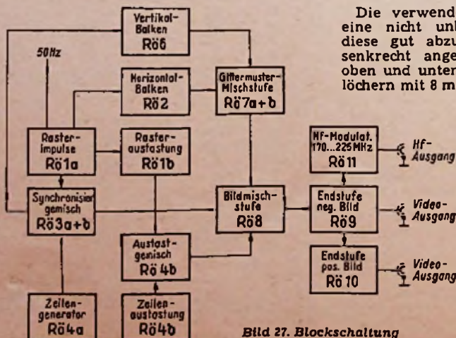
Bild 27. Blockschaltung
