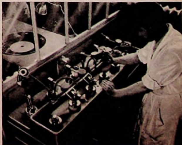
Rechts: Die Spezialmaschine, auf der Glaskolben und Preßsteller genau aufeinanderpassend geläpft (feingeschliffen) werden. Links im Bild sind drei Lüppvorrichtungen für Preßsteller, rechts drei ebensolche für Glaskolben zu sehen
