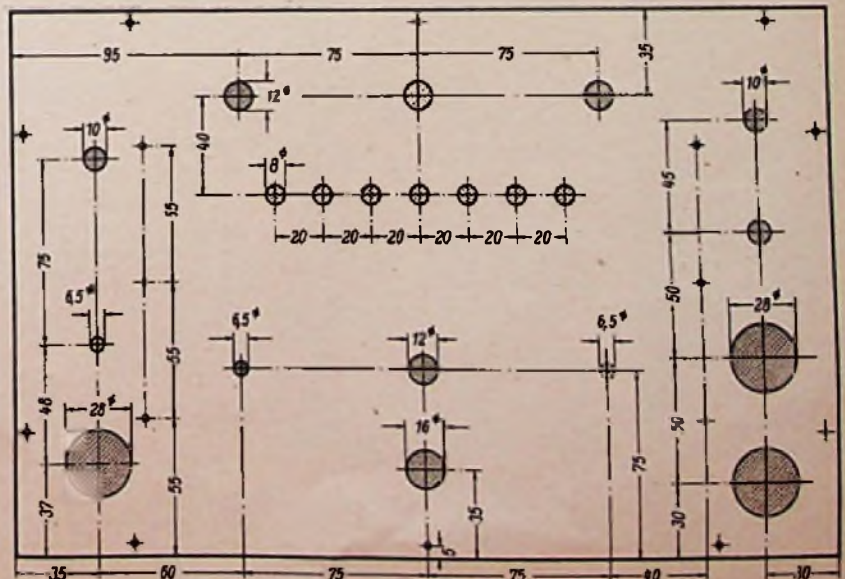
Bild 10. Chassis, Eisenblech, 1,5 mm stark
