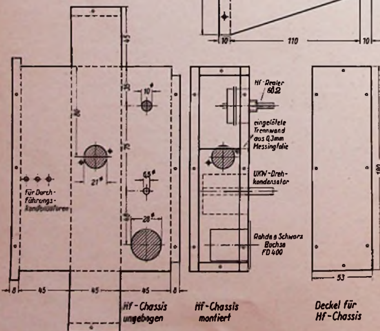
Bild 6. Teile für den Hf-Baustein. Werkstoff: Messingblech 1 mm
