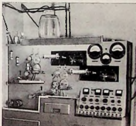
Maschine, auf der in kontinuierlichem Prozeß die Drähte für Gitter, Halterung usw. vergoldet werden. Die Stärke der Vergoldung wird auf Bruchteile von \mu eingehalten. Die Vergoldung aus solche ist ein bekanntes Verfahren und hat den Sinn, die Elektronenaustrittsarbeit zu vergrößern
