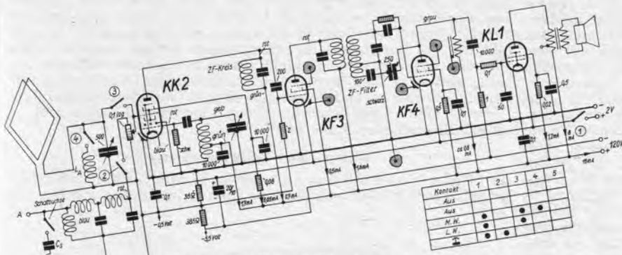
Die Gesamtschaltung des Wander-Super. Die Spulen La und Ls sind selbst gewickelt. La mit 72 Windungen 20 \times 0,05 und Ls mit 110 Windungen 20 \times 0,05 , beide auf Ferrocarril-Topfkern mit vergrößertem Abgleichbereich. Zwischen dem Anschluß A (Antenne) und E (Erde) der aus Cs und Ls bestehende Saugkreis.
